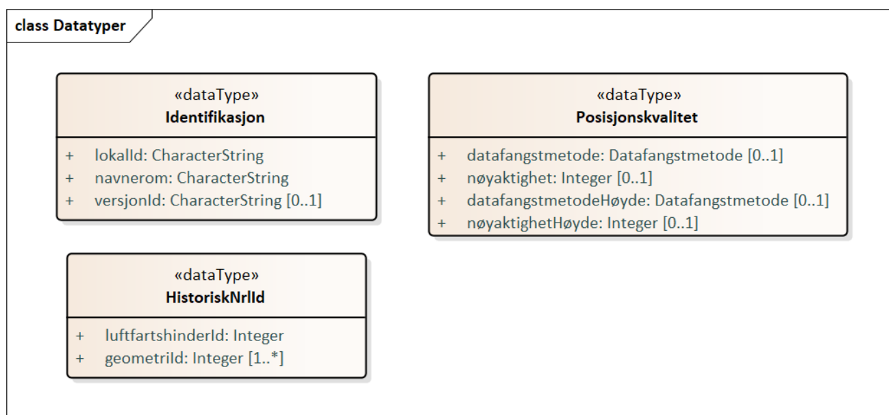
Figur 8. Datatyper
