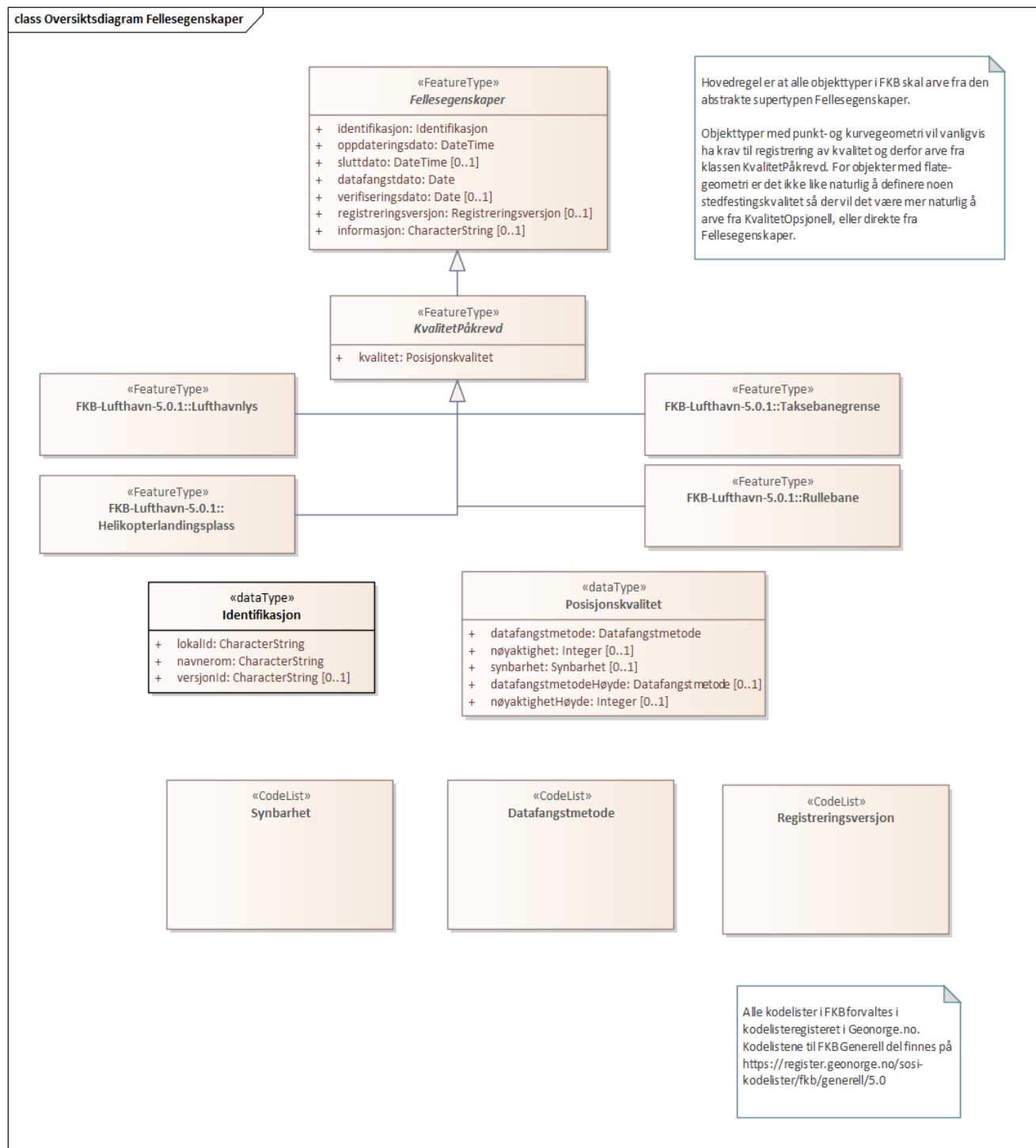
Figur 8. Oversiktsdiagram Fellesegenskaper
