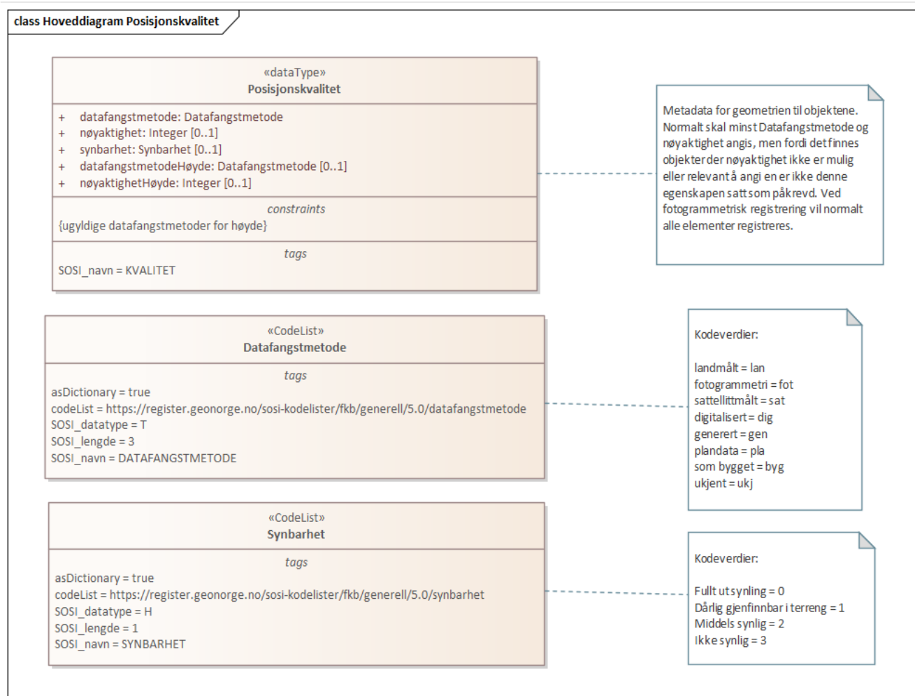
Figur 10. Hoveddiagram Posisjonskvalitet
