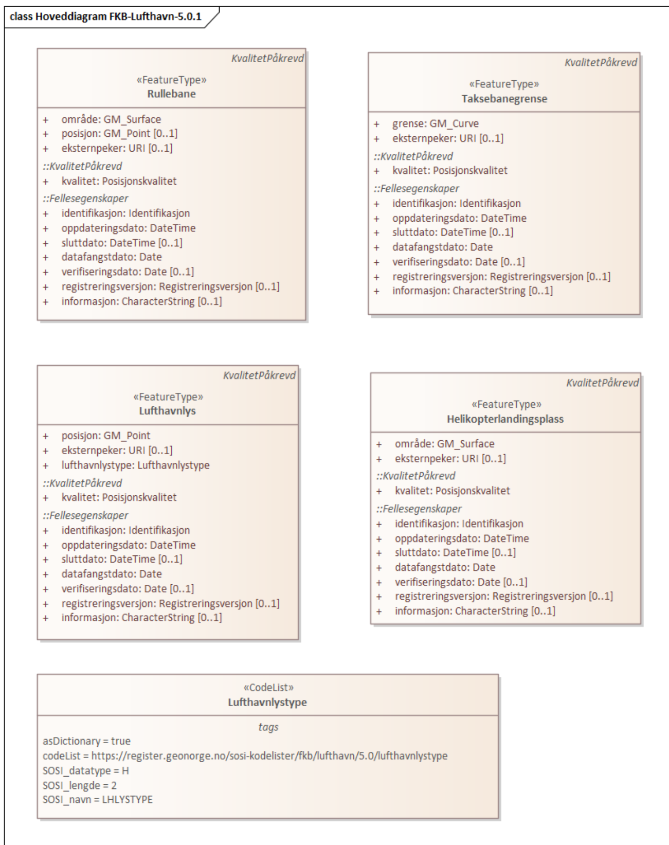
Figur 2. Hoveddiagram FKB-Lufthavn-5.0.1
