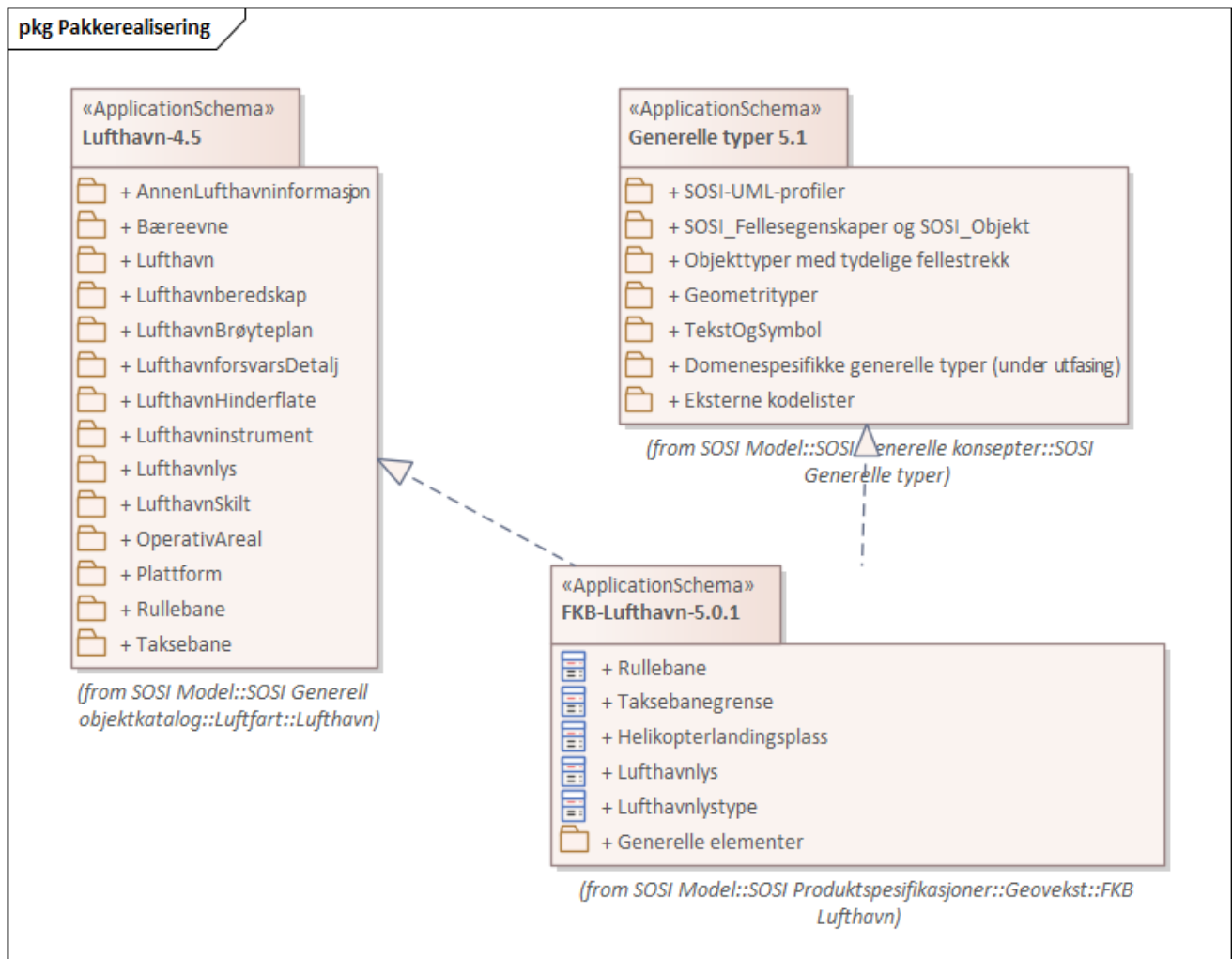
Figur 1. Pakkerealisering
