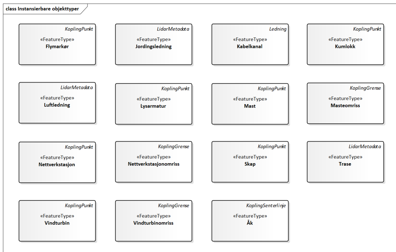
Figur 5. Instansierbare objekttyper
