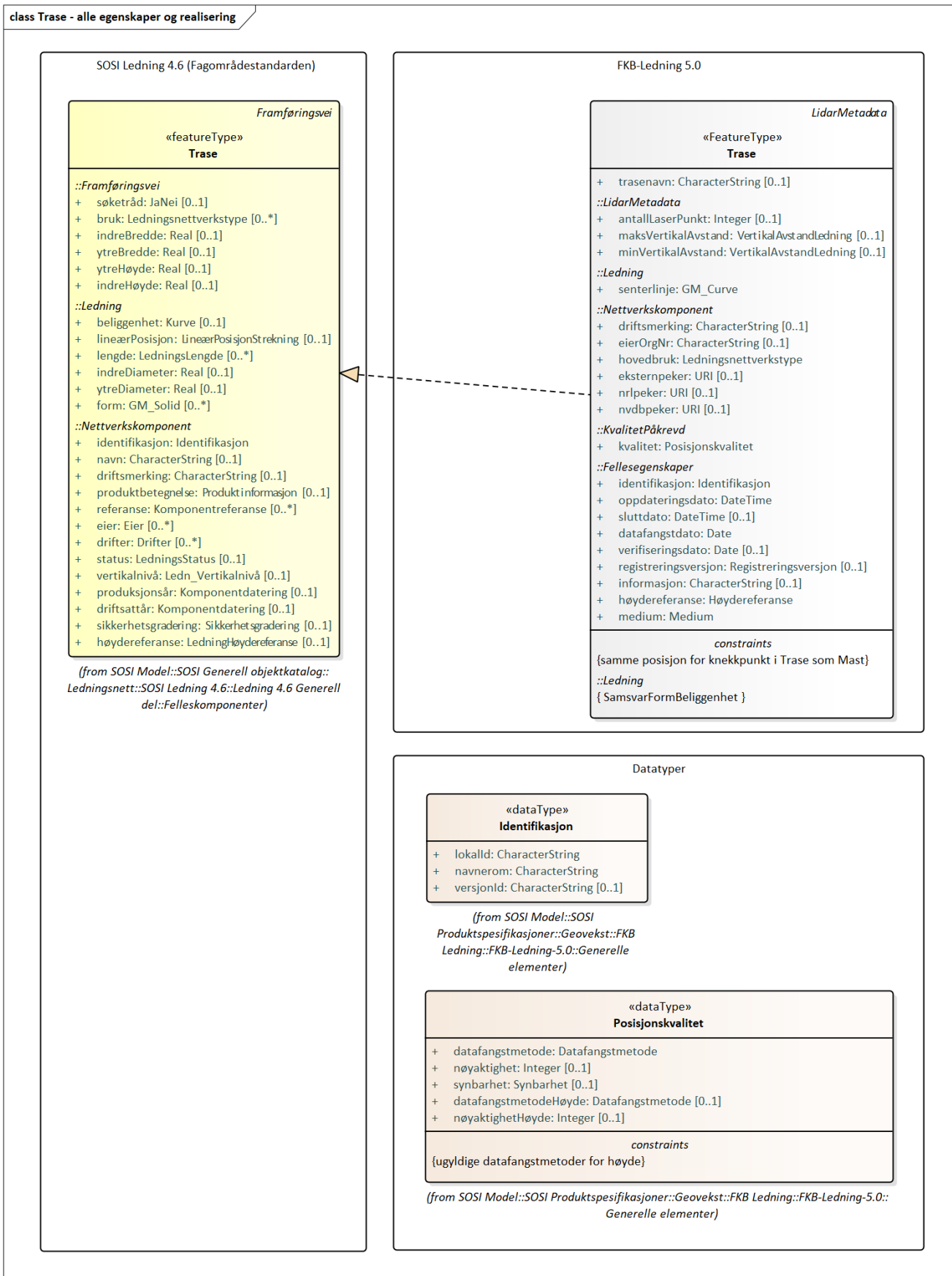
Figur 15. Trase - alle egenskaper og realisering
