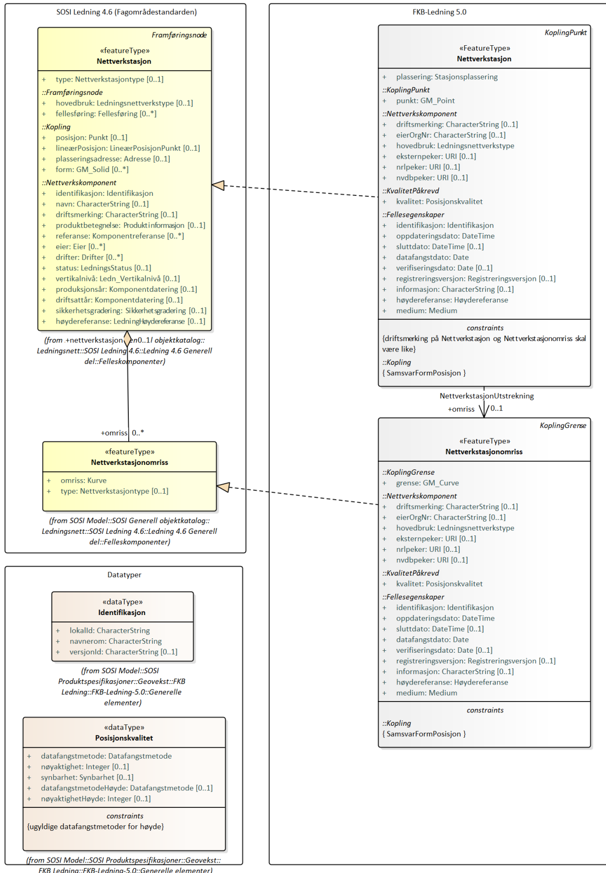
Figur 13. Nettverkstasjon og Nettverkstasjonomriss - alle egenskaper og realisering
