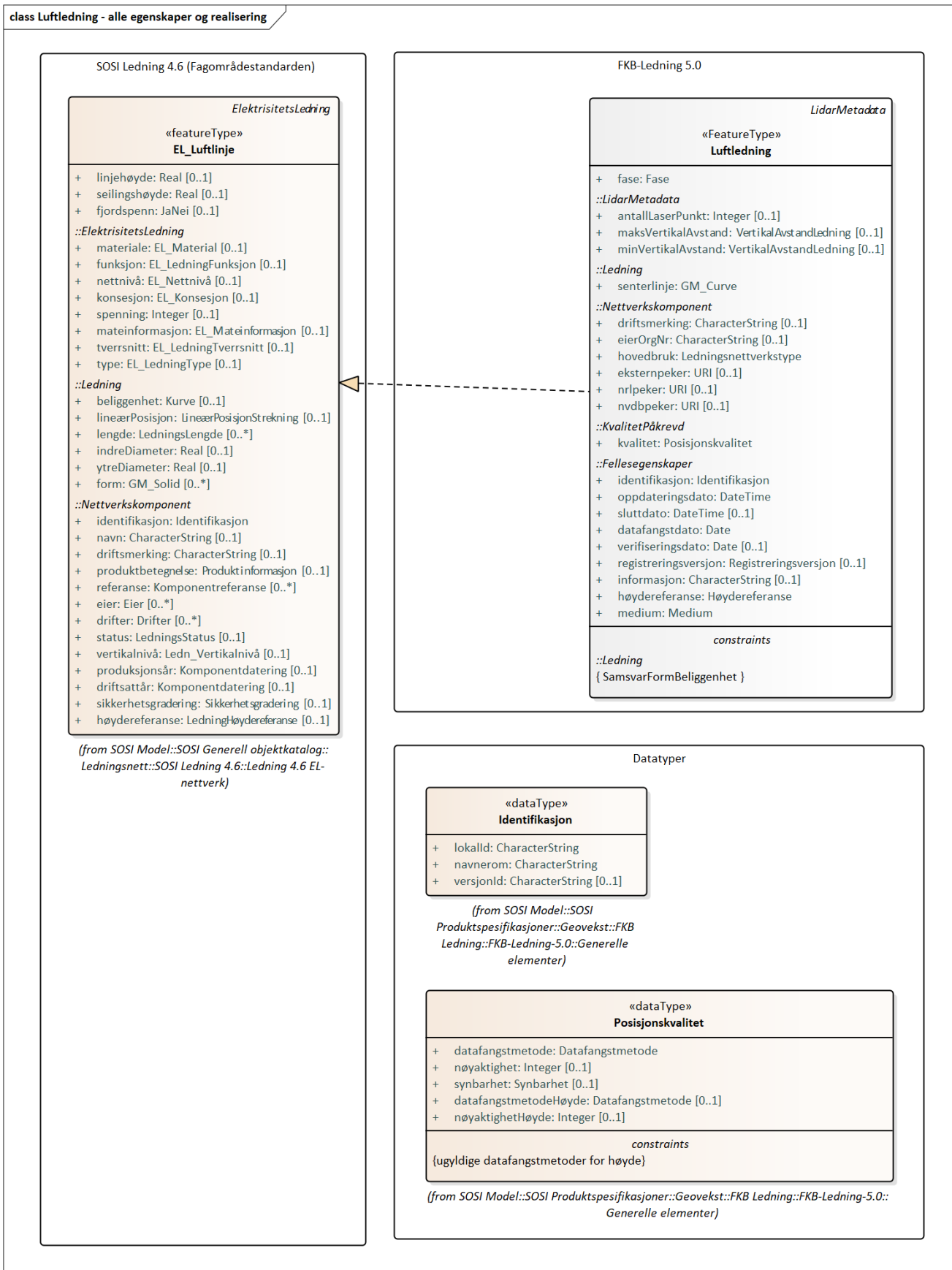
Figur 10. Luftledning - alle egenskaper og realisering
