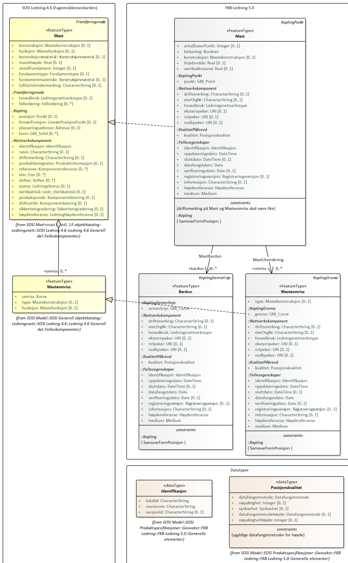
Figur 12. Mast Masteomriss og Bardun - alle egenskaper og realisering
