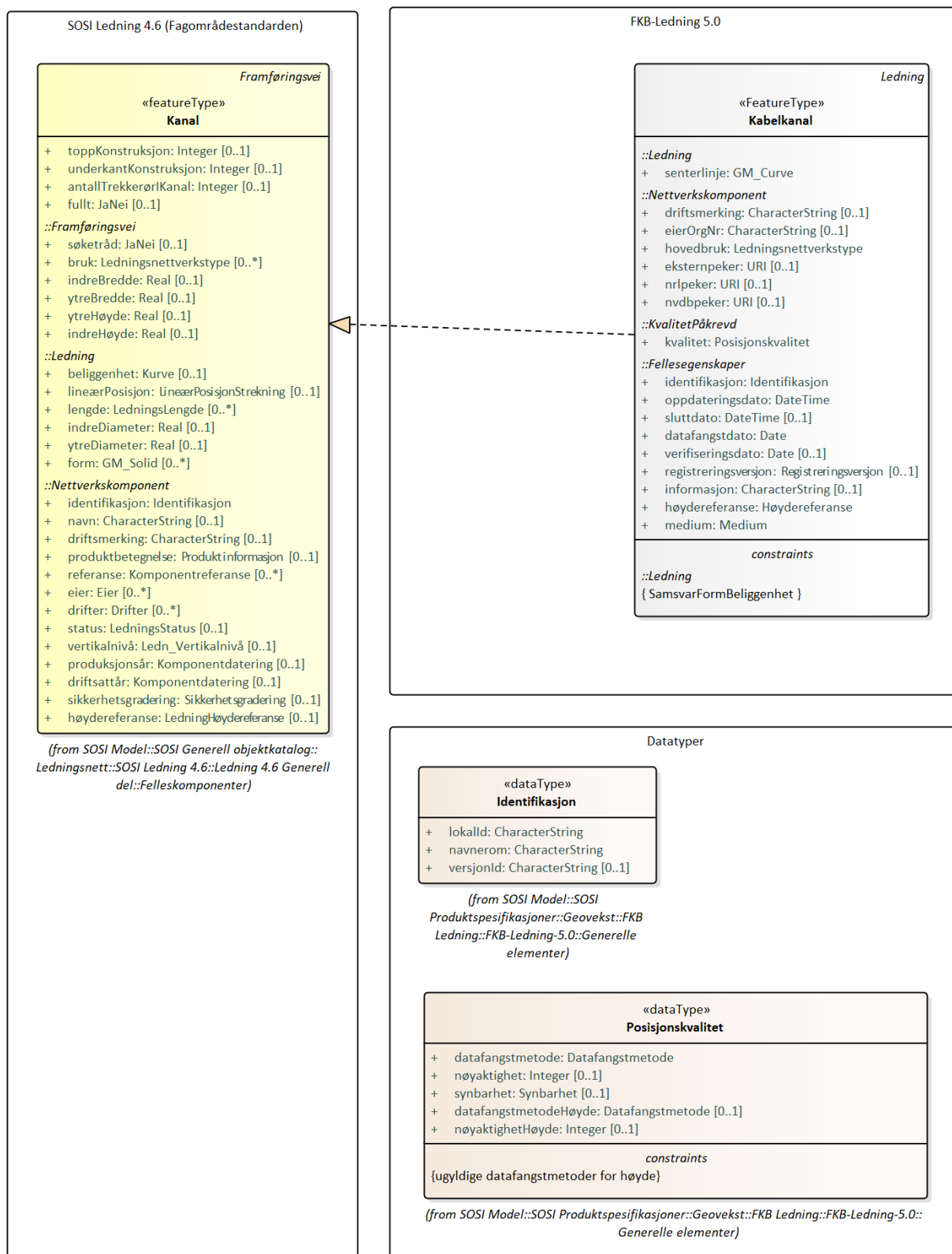
Figur 8. Kabelkanal - alle egenskaper og realisering
