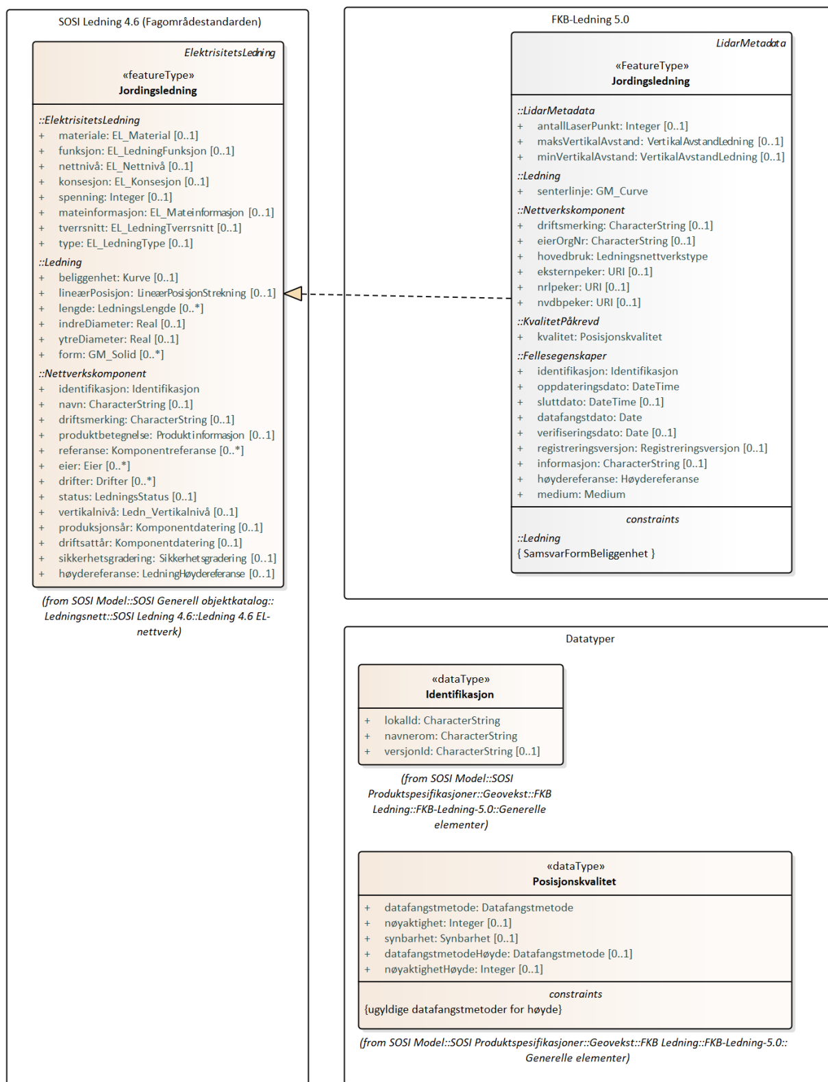
Figur 7. Jordingsledning - alle egenskaper og realisering
