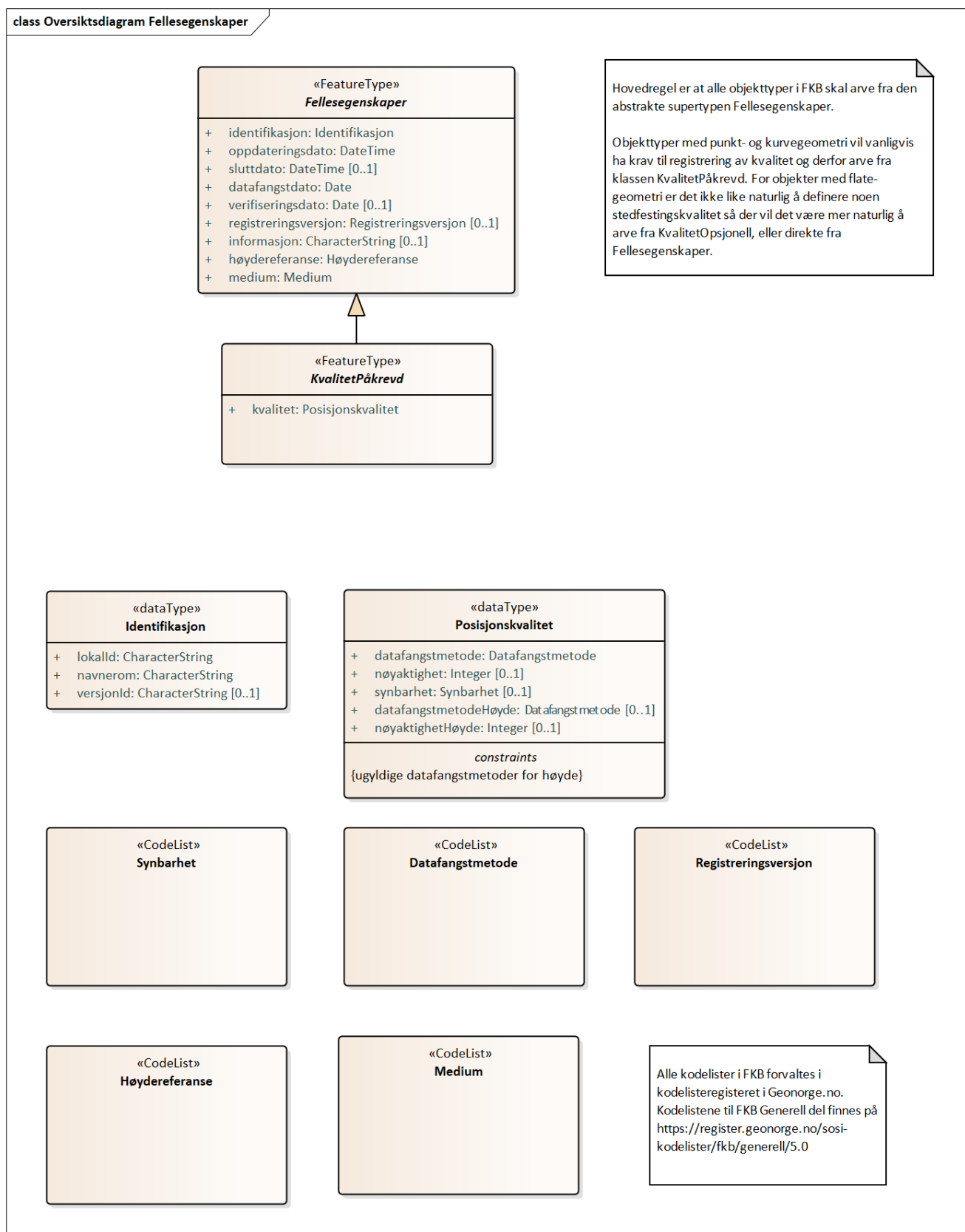
Figur 35. Oversiktsdiagram Fellesegenskaper
