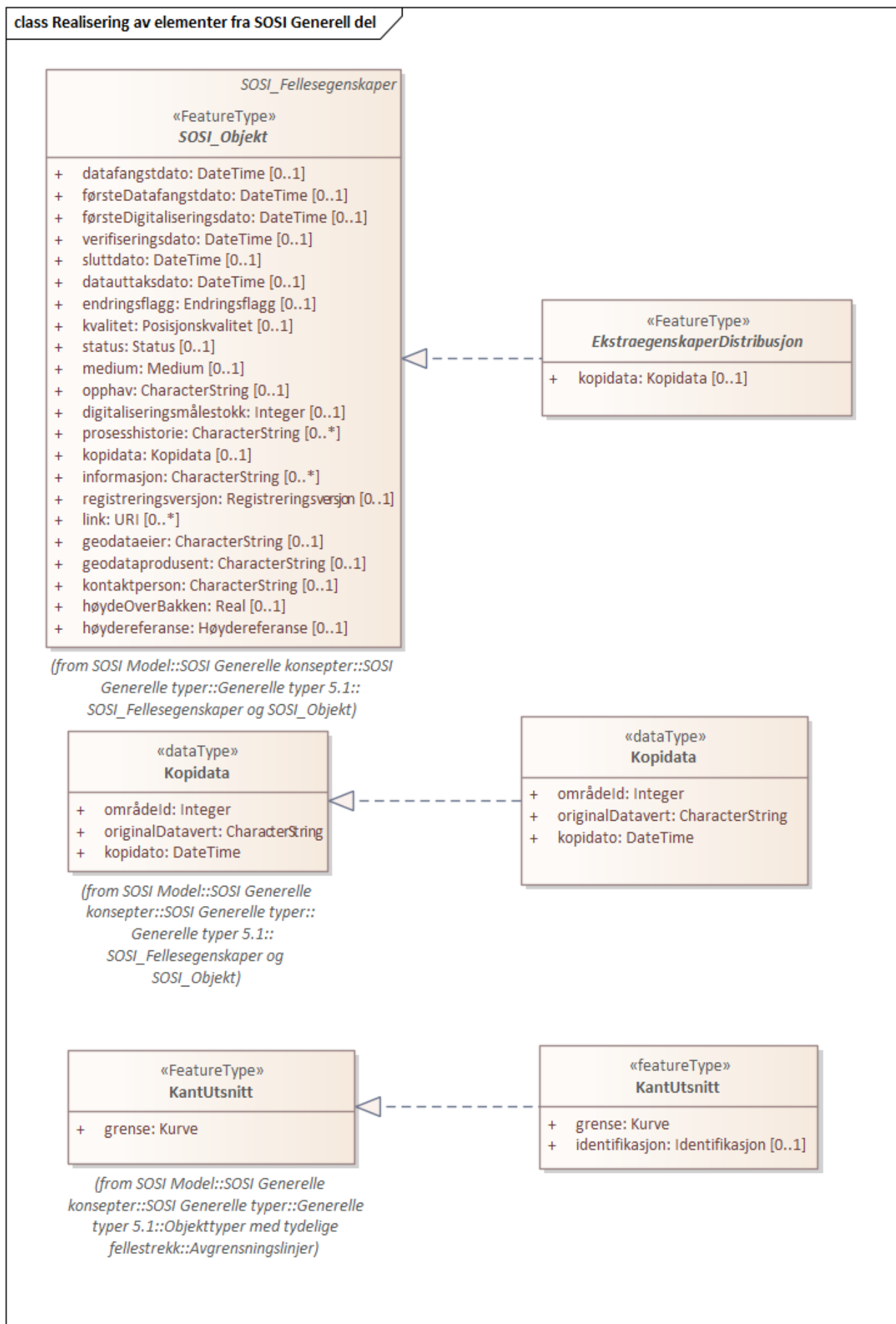
Figur 15. Realisering av elementer fra SOSI Generell del
