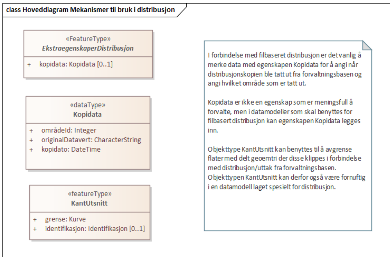
Figur 14. Hoveddiagram Mekanismer til bruk i distribusjon
