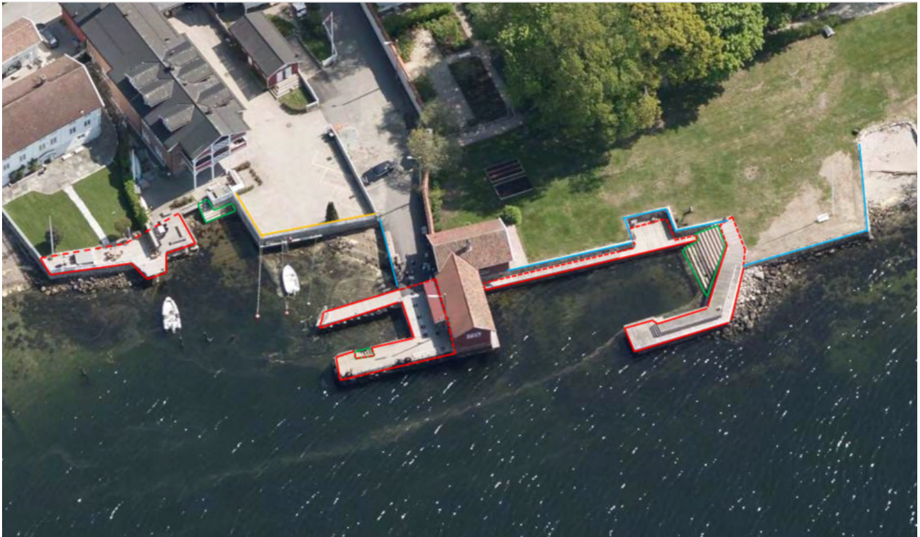
Figur 76. Eksempel på registrering av KaiBryggekanth (rød helstrek), FiktivAvgrensningForAnlegg (rød stiplet), MurLoddrett (blått), AnnetGjerde (gult), Trapp (grønt).
