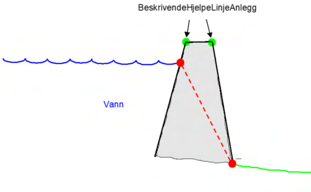
Figur 62. Skisse som viser høydereferanse for registrering av demning. Demningens avgrensning registreres som de røde objektene. Toppen av Demning registreres med BeskrivendeHjelpelinjeAnlegg
