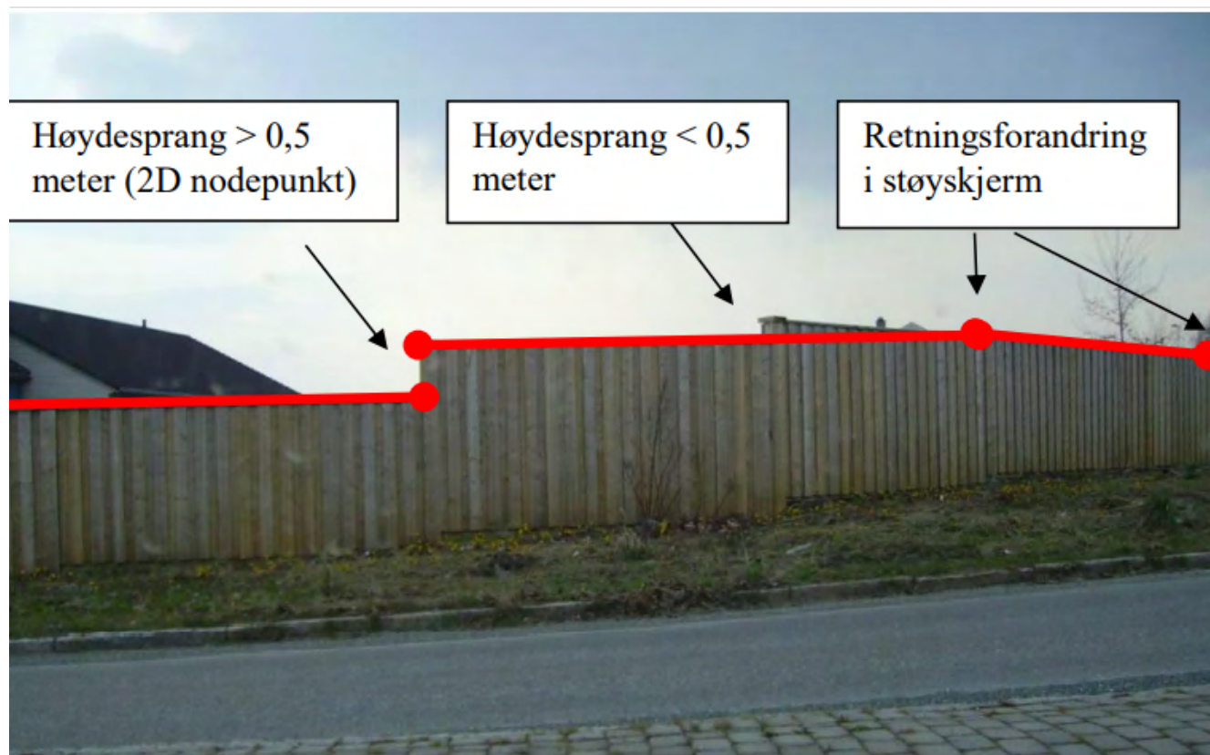
Figur 36. Eksempel på registrering av støyskjerm. Det lages 2D nodepunkt der det er høydesprang på mer enn 0.5 meter. Samme prinsipp for høyderegistrering gjelder også for veldig mange andre objekttyper i FKB-BygnAnlegg som Gjerde etc.
