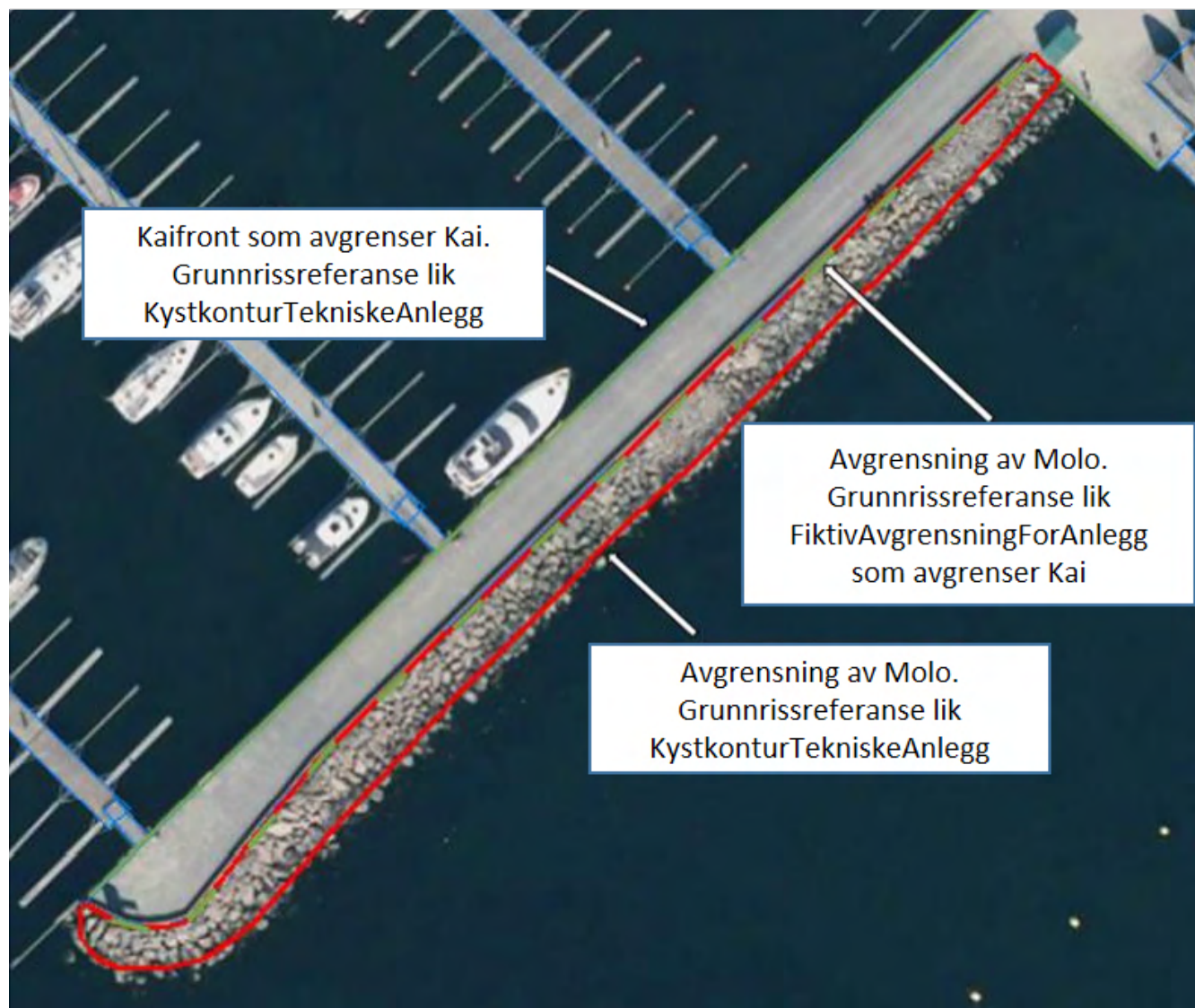
Figur 79. Eksempel på registrering av situasjon der Molo ligger inntil Kai
