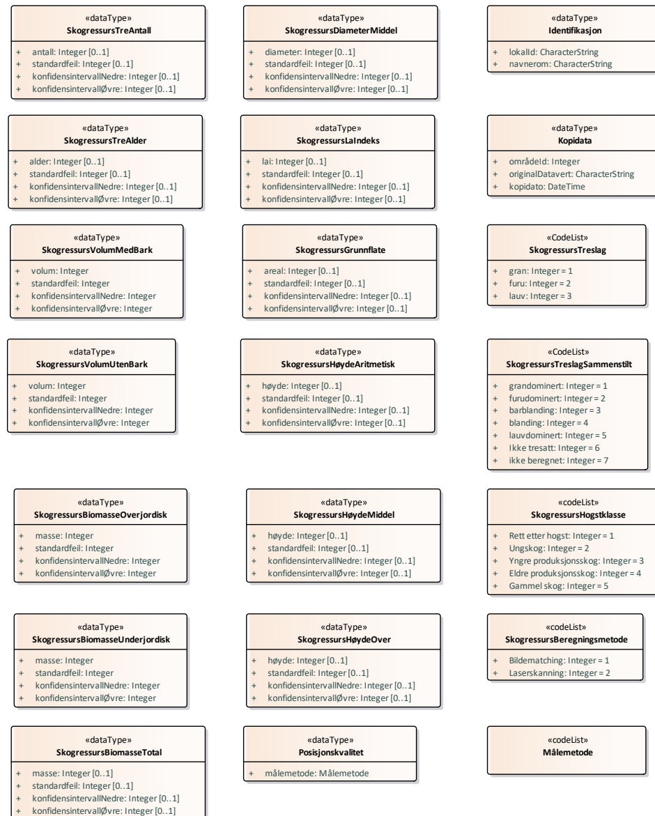
Figur 5 Datatyper og kodelister
