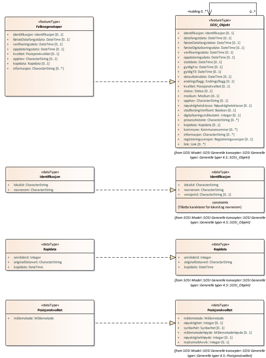
Figur 3 Realiseringer fra SOSI-objekt
