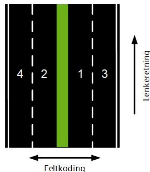
Figur 4: Feltkoden gir oss informasjon om kjørefeltene i vegens tverrsnitt.
