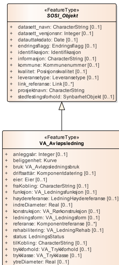
Figur 17: Hoveddiagram: VA_Avløpsledning
