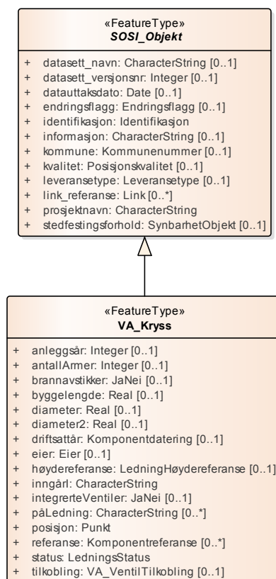
Figur 31: Hoveddiagram: VA_Kryss
