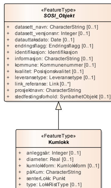
Figur 9: Hoveddiagram: Kumlokk
