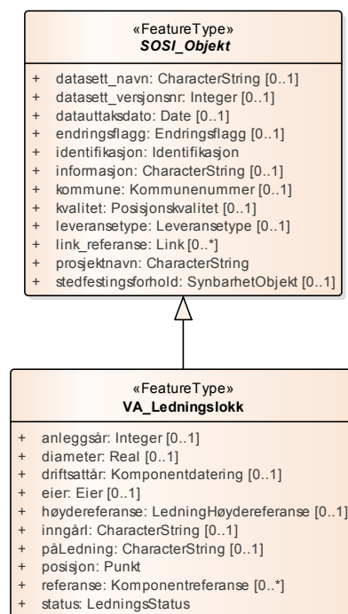
Figur 35: Hoveddiagram: VA_Ledningslokk
