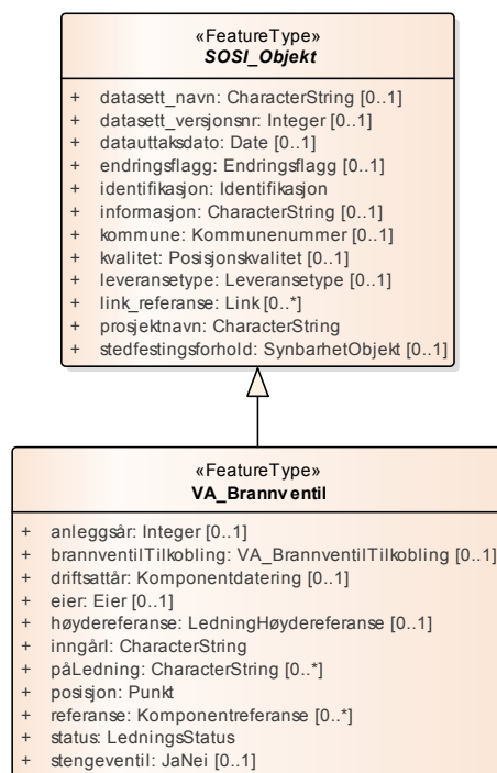
Figur 25: Hoveddiagram: VA_Brannventil
