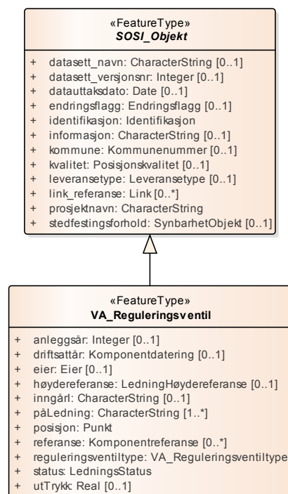
Figur 51: Hoveddiagram: VA_Reguleringsventil
