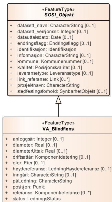
Figur 23: Hoveddiagram: VA_Blindflens
