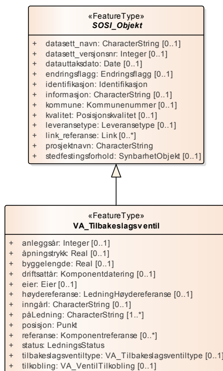
Figur 55: Hoveddiagram: VA_Tilbakeslagsventil
