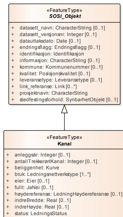
Figur 5: Hoveddiagram: Kanal
