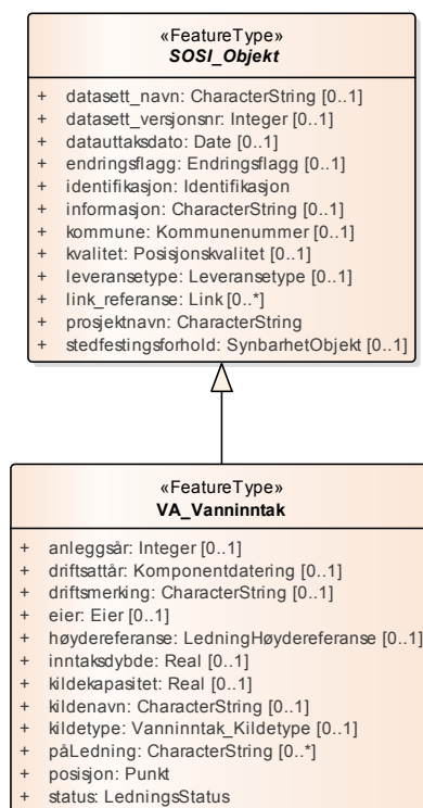
Figur 61: Hoveddiagram: VA_Vanninntak
