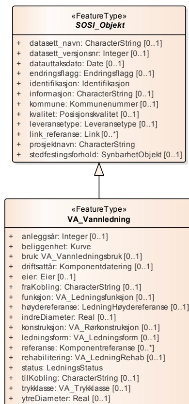
Figur 63: Hoveddiagram: VA_Vannledning
