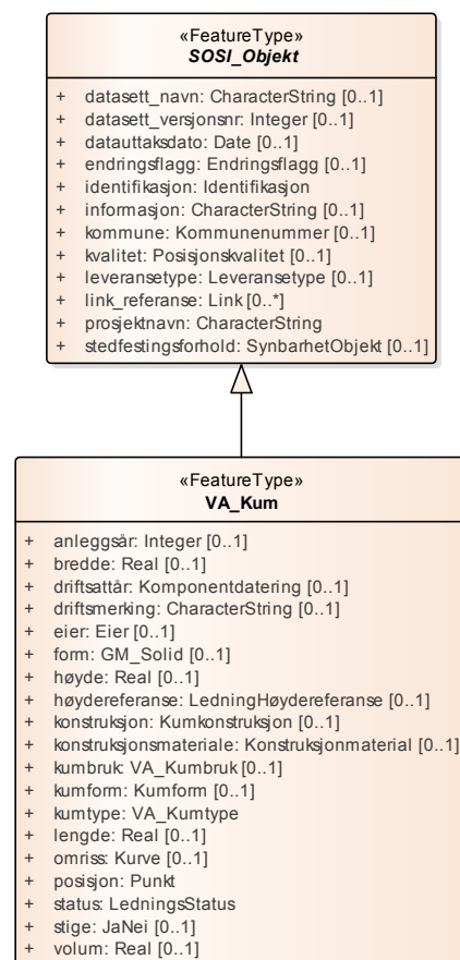
Figur 33: Hoveddiagram: VA_Kum
