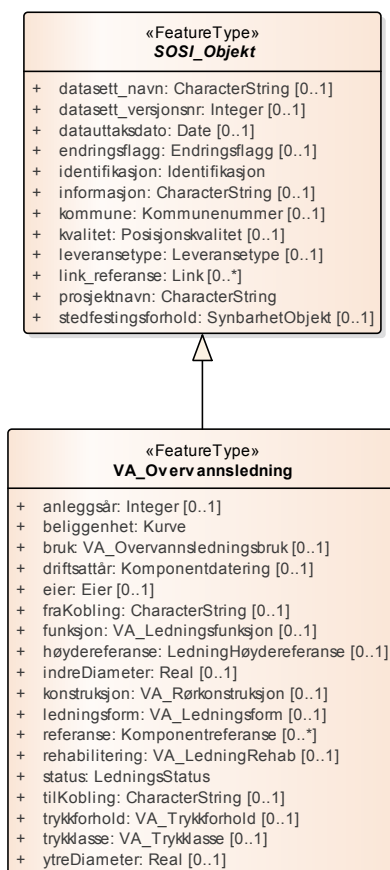
Figur 47: Hoveddiagram: VA_Overvannsledning
