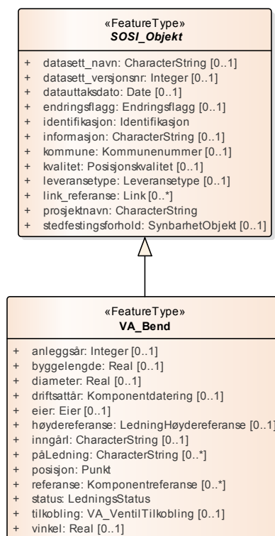
Figur 21: Hoveddiagram: VA_Bend
