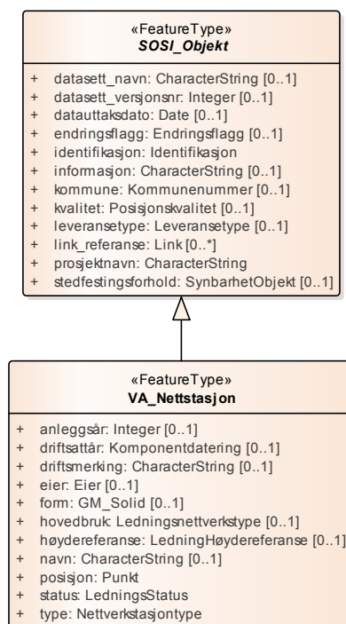
Figur 43: Hoveddiagram: VA_Nettstasjon
