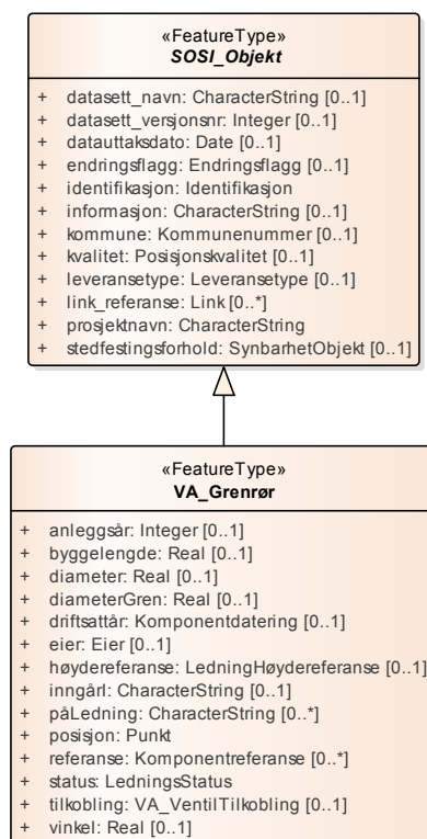
Figur 27: Hoveddiagram: VA_Grennrør
