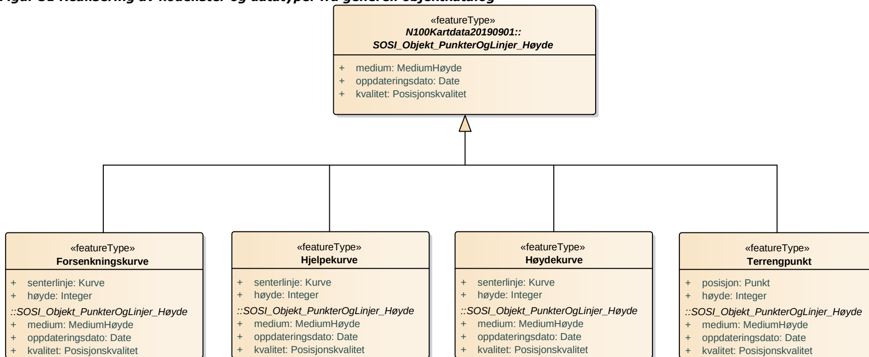
Figur 31 Realisering av kodelister og datatyper fra generell objektkatalog
