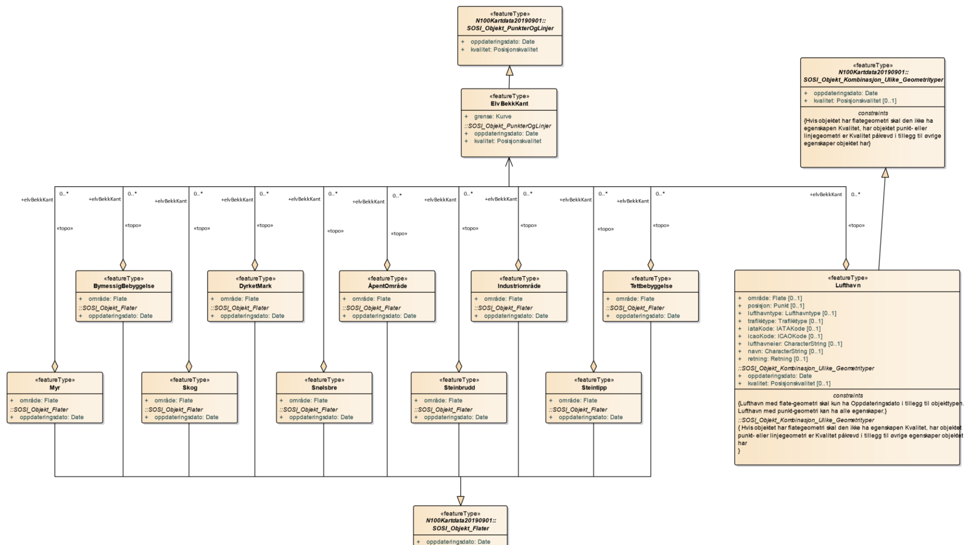
Figur 15 Arealdekke_ElvBekkKant
