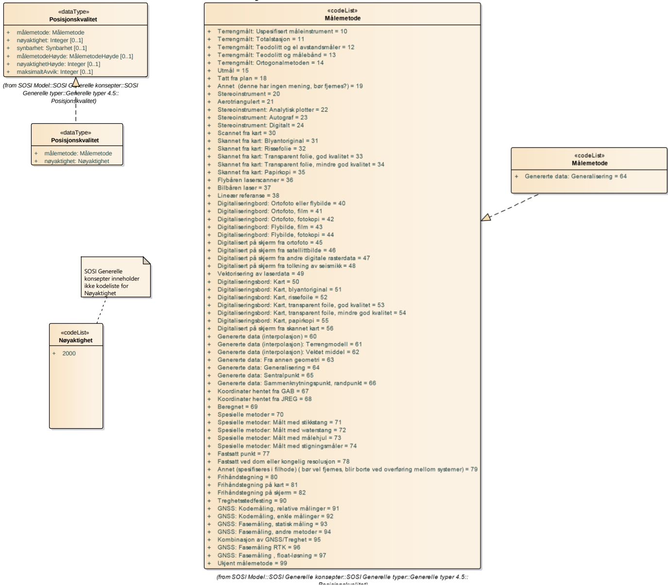
Figur 3 Posisjonskvalitet
