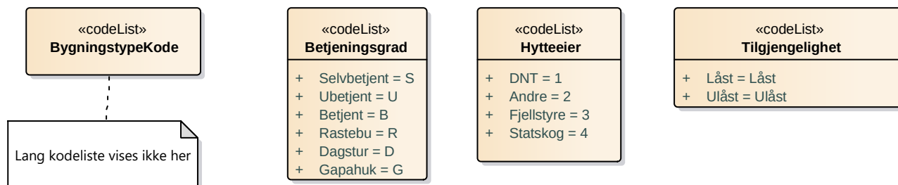
Figur 28 Kodelister
