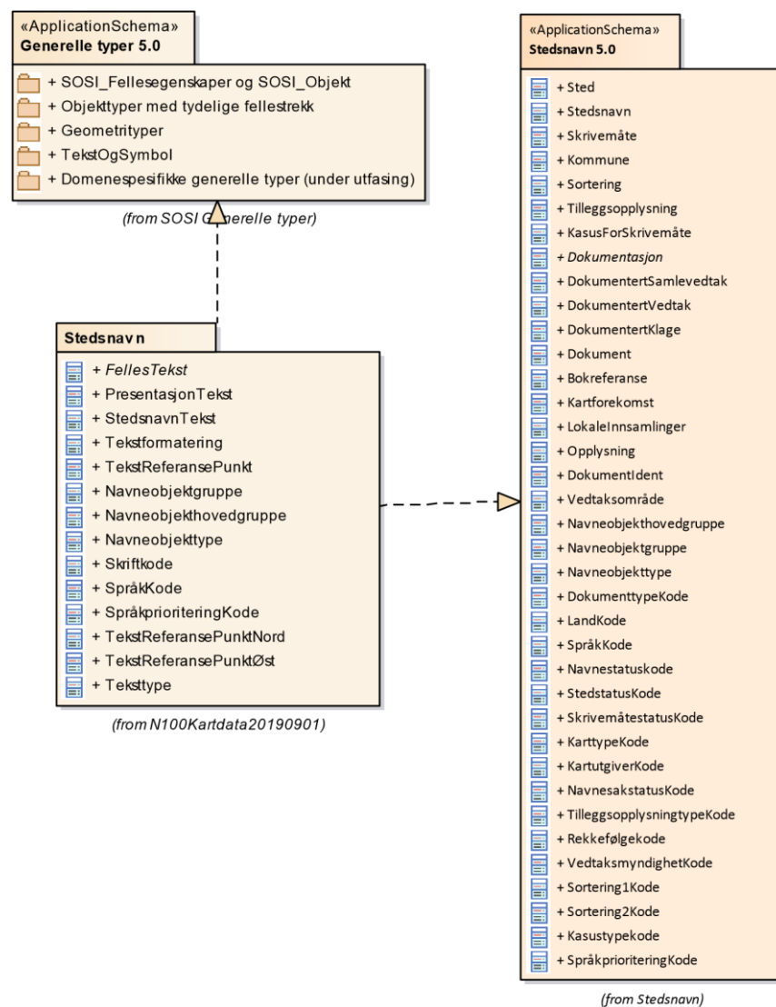
Figur 46 Pakkeavhengighet
