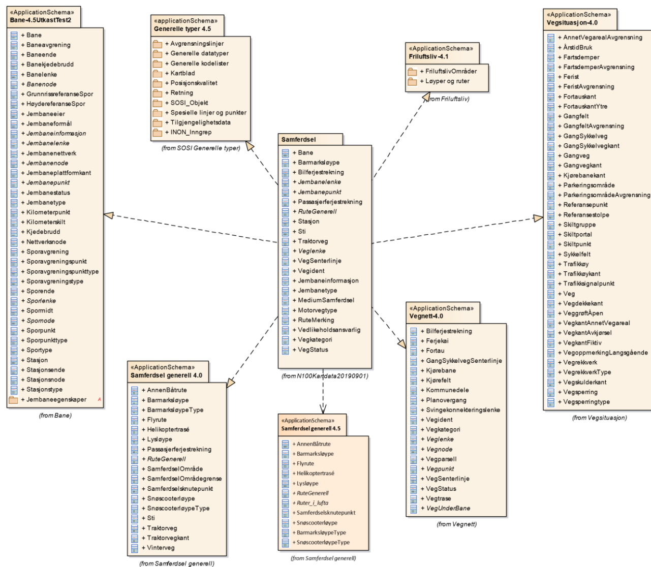
Figur 39 Pakkeavhengighet
