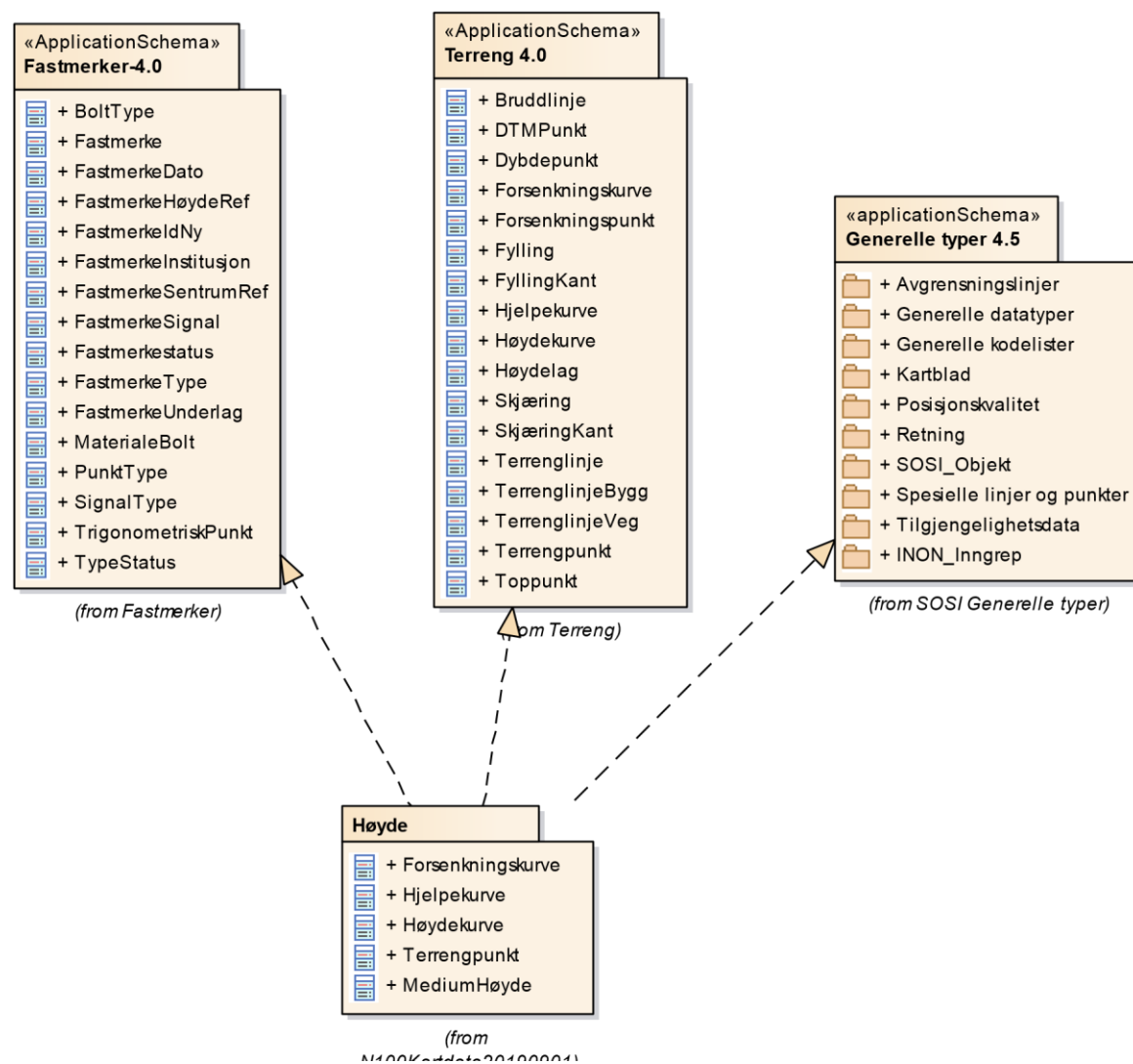
Figur 29 Pakkeavhengighet
