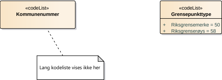
Figur 9 Kodeliste
