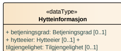
Figur 27 Datatyper
