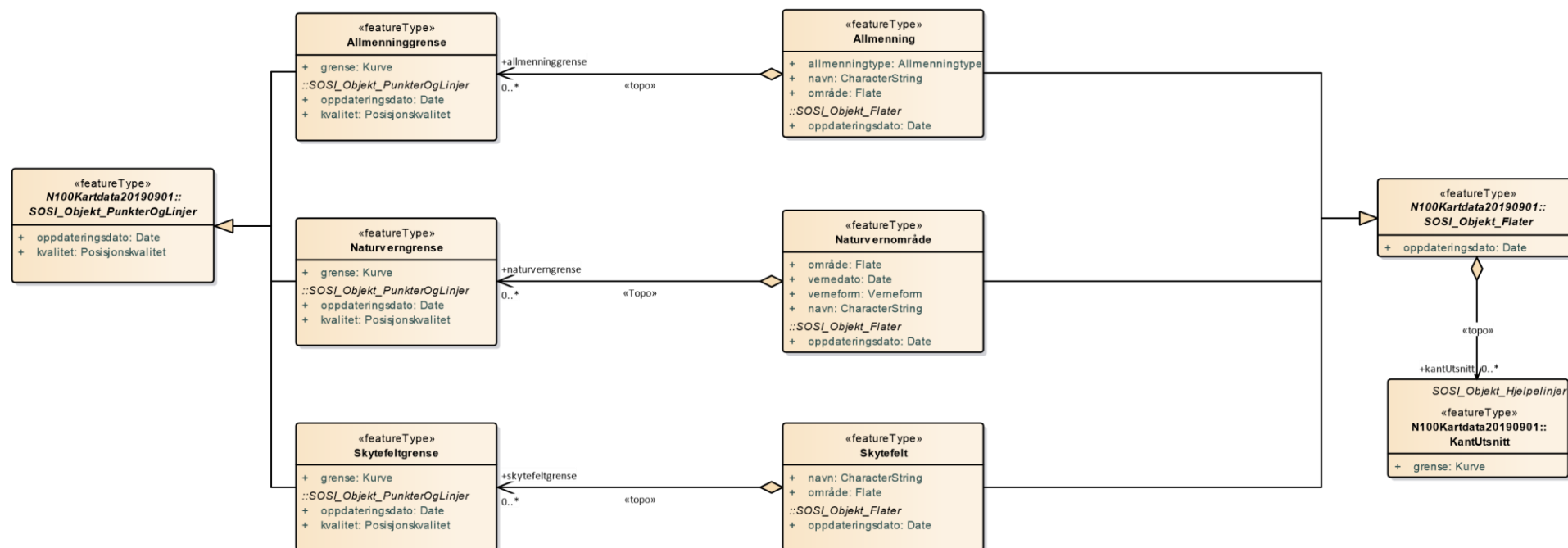
Figur 37 Restriksjonsområder
