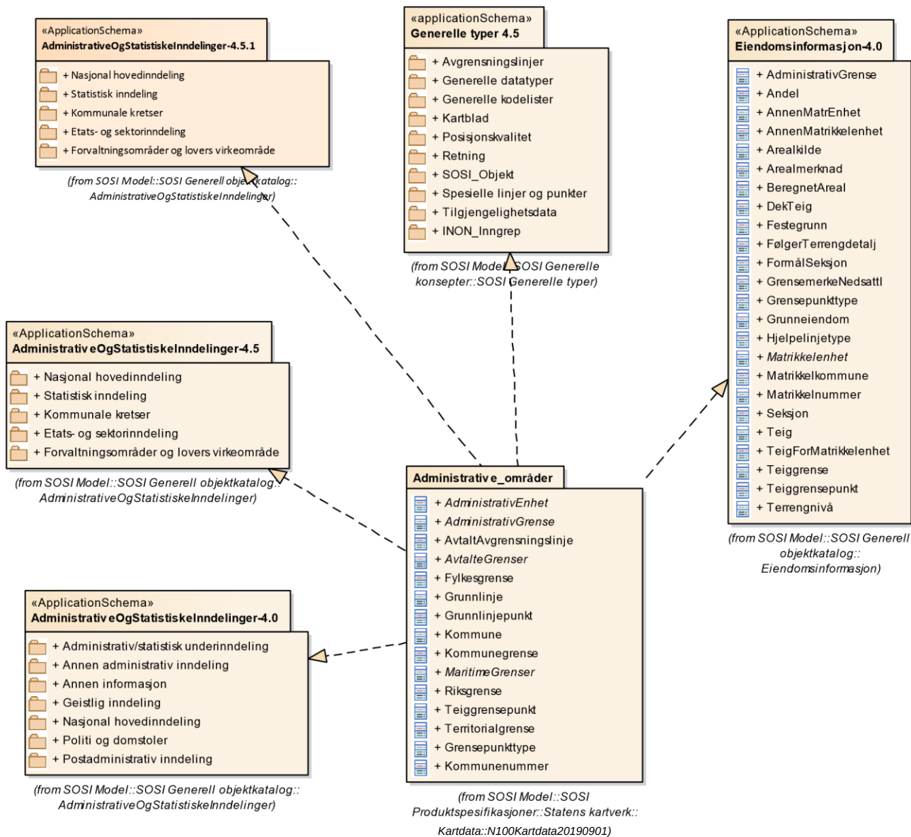
Figur 5 Pakkeavhengighet
