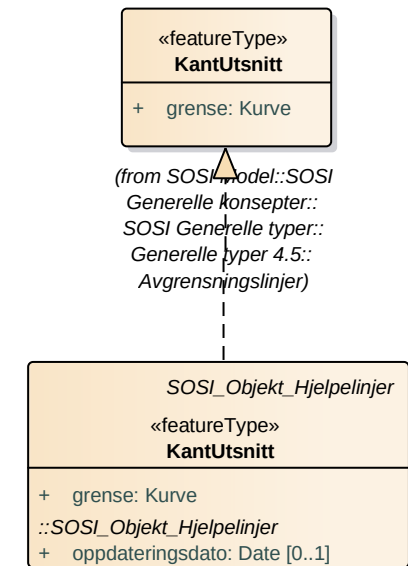
Figur 2 KantUtsnittrealisering
