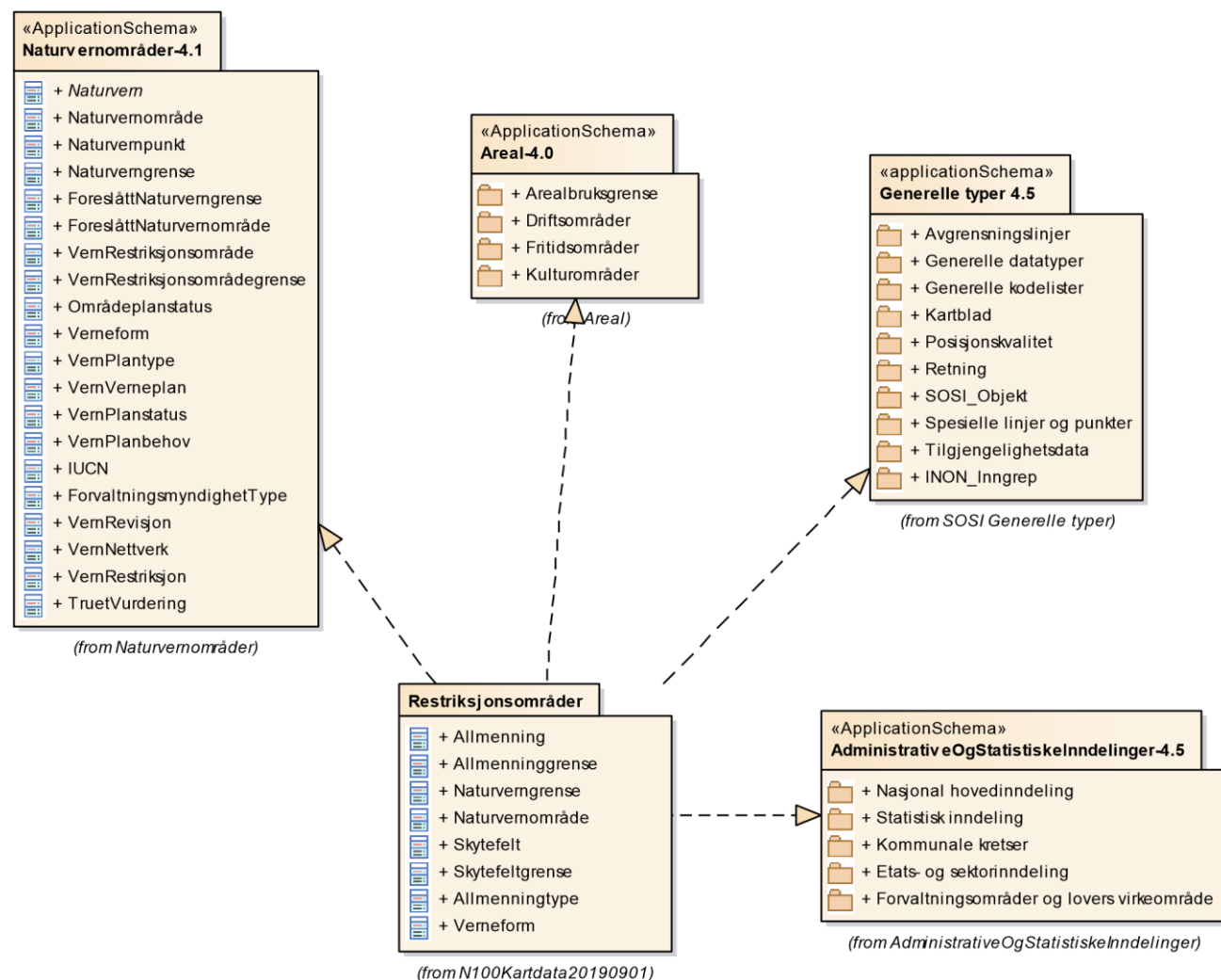
Figur 34 Pakkeavhengighet
