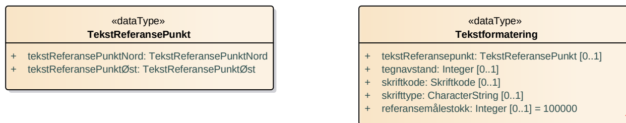
Figur 50 Datatyper
