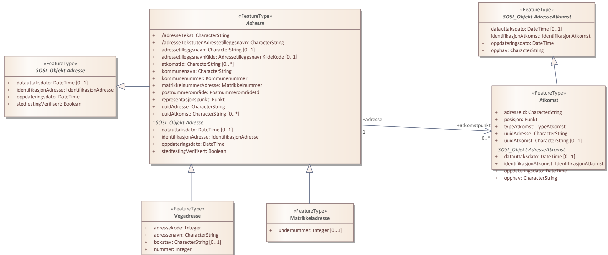
Figur 1: Hoveddiagram Matrikkelen-Vegadresse
