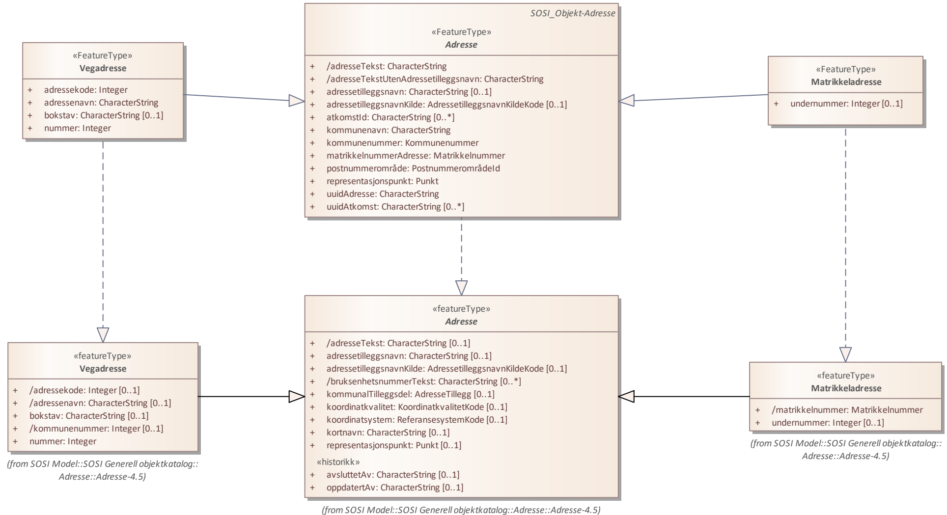
Figur 2: Realisering Objekttyper
