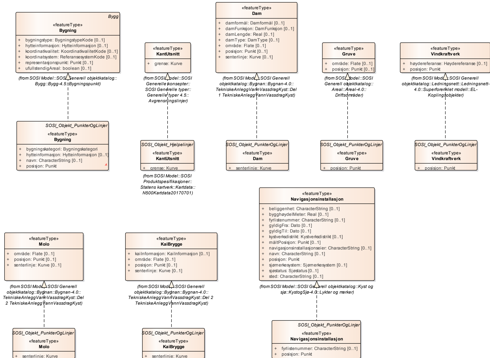
Figur 24 Realisering av featuretyper fra generell objektkatalog
