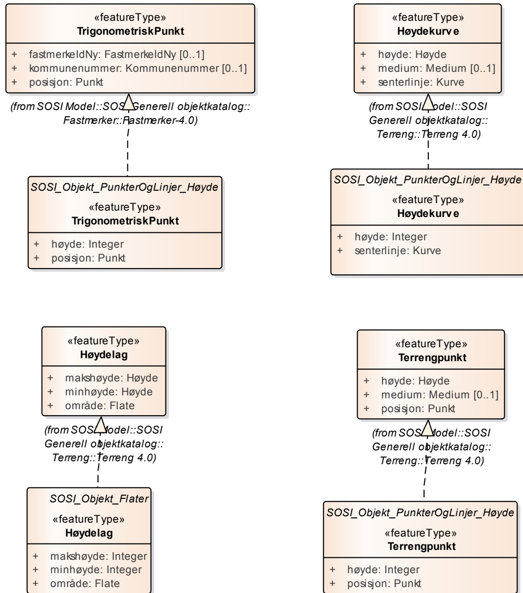
Figur 31 Realisering av featuretyper fra generell objektkatalog
