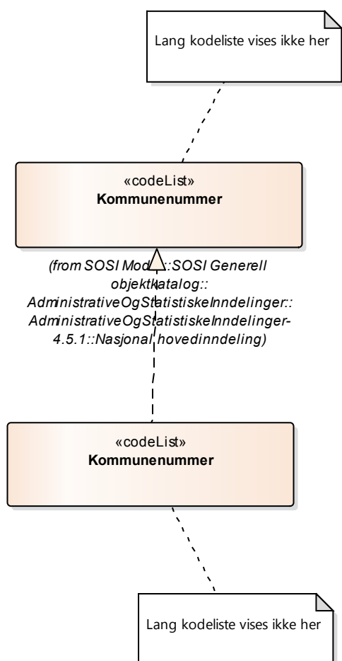
Figur 8 Realisering av kodelister fra generell objektkatalog
