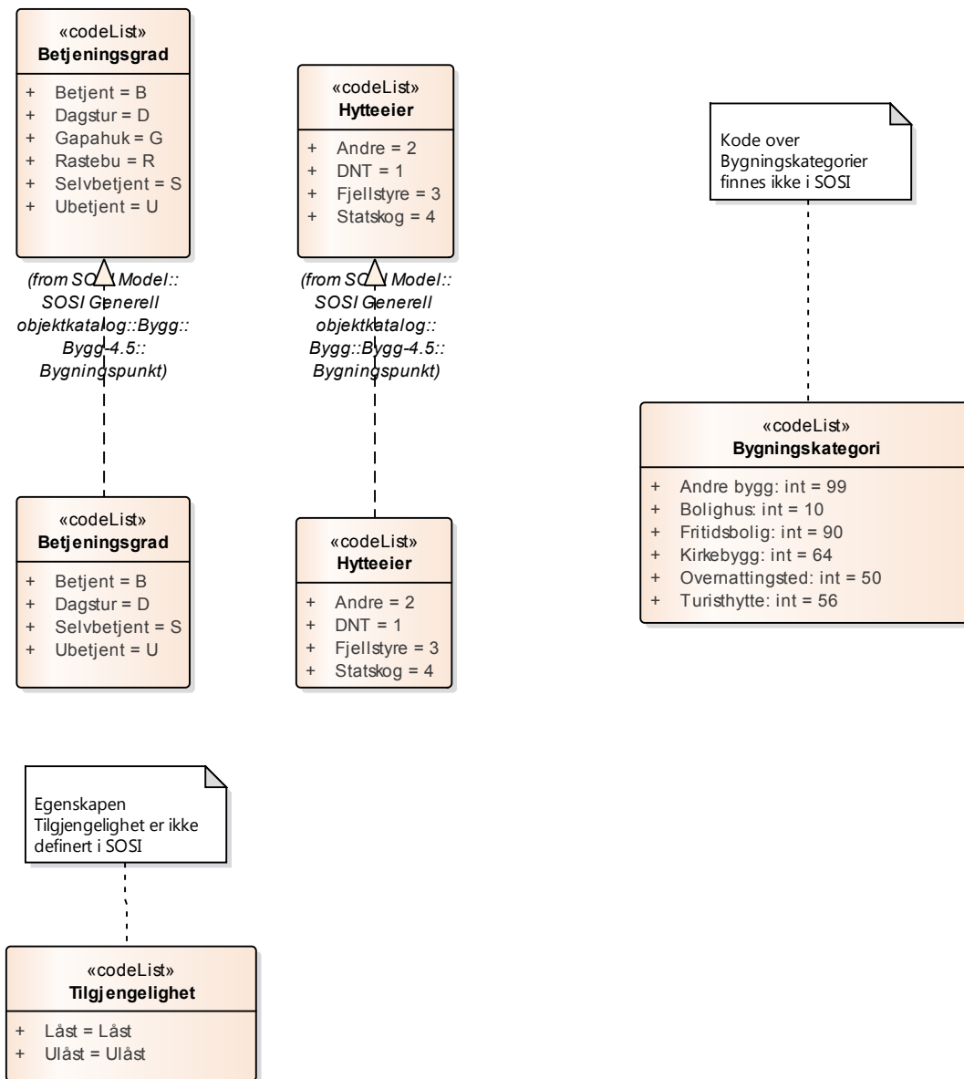
Figur 26 Realisering av kodelister fra generell objektkatalog
