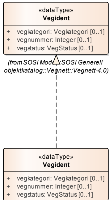
Figur 43 Realisering av datatyper fra generell objektkatalog
