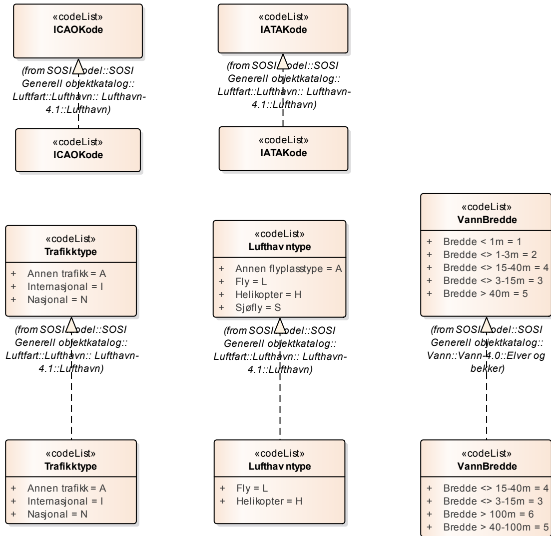
Figur 14 Realisering av kodelister fra generell objektkatalog
