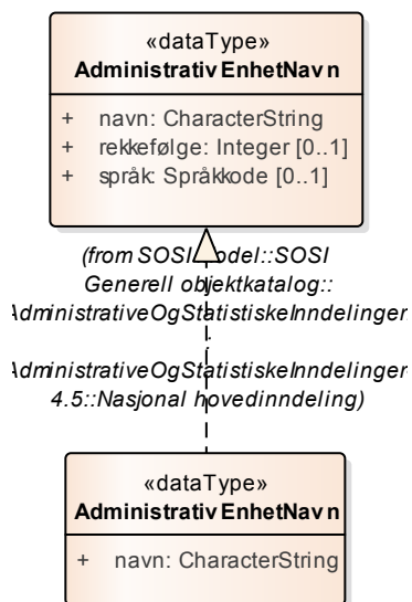
Figur 7 Realisering av datatyper fra generell objektkatalog
