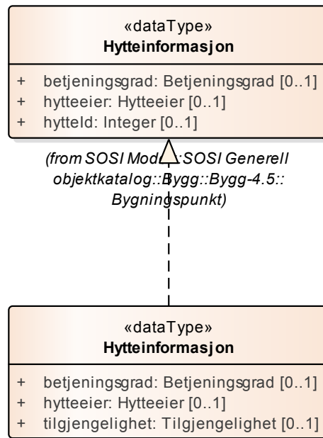
Figur 25 Realisering av datatyper fra generell objektkatalog
