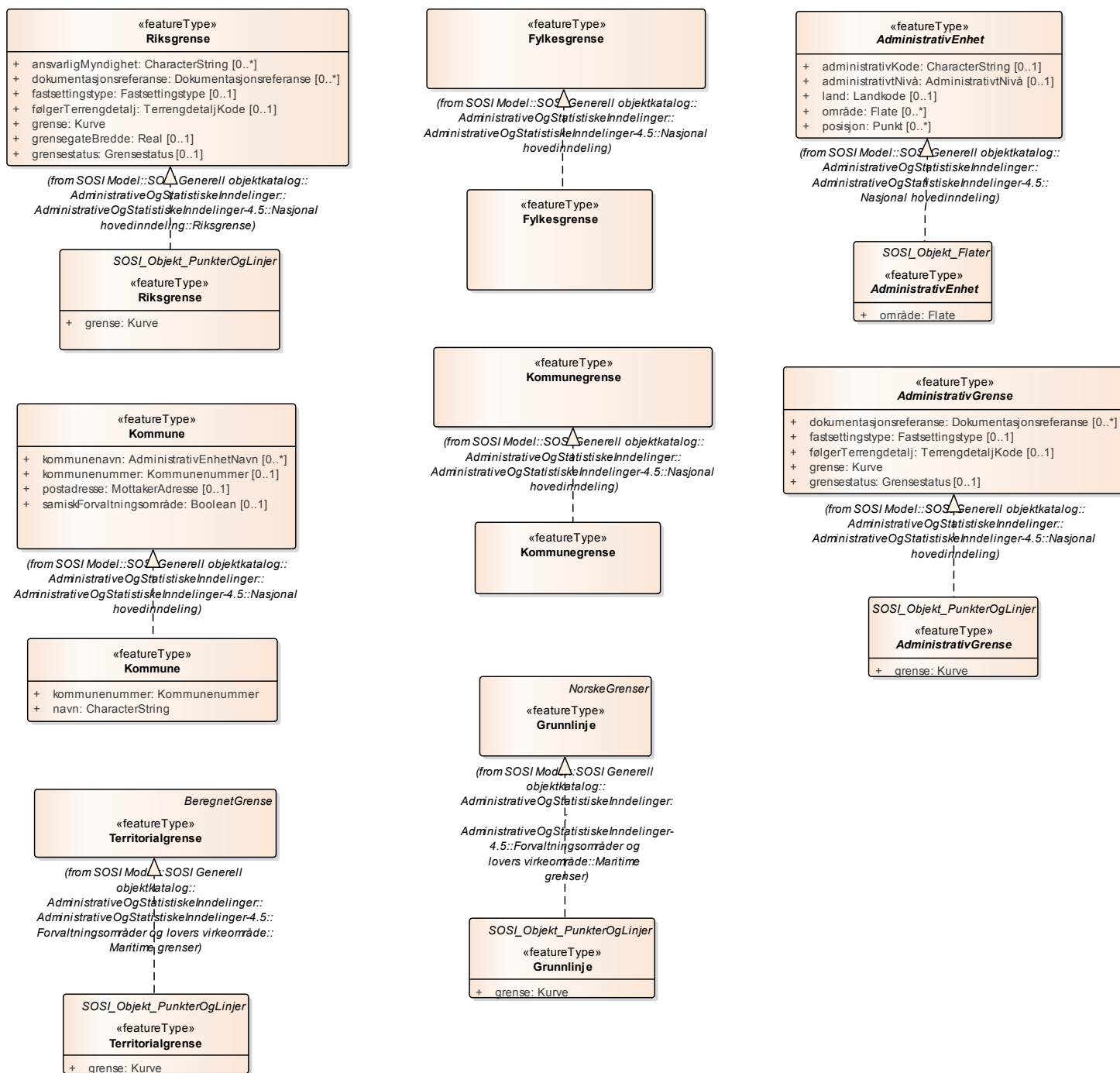
Figur 6 Realisering av featuretyper fra generell objektkatalog
