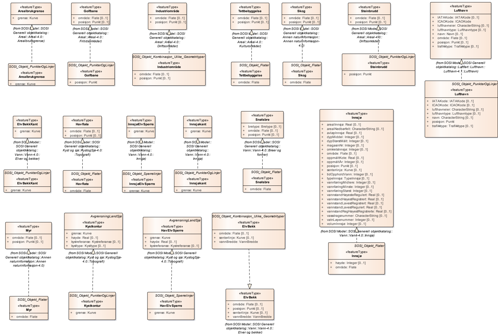
Figur 13 Realisering av featuretyper fra generell objektkatalog
