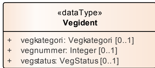
Figur 42 Datatyper
