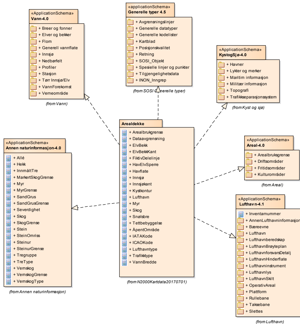
Figur 12 Pakkerealiserings
