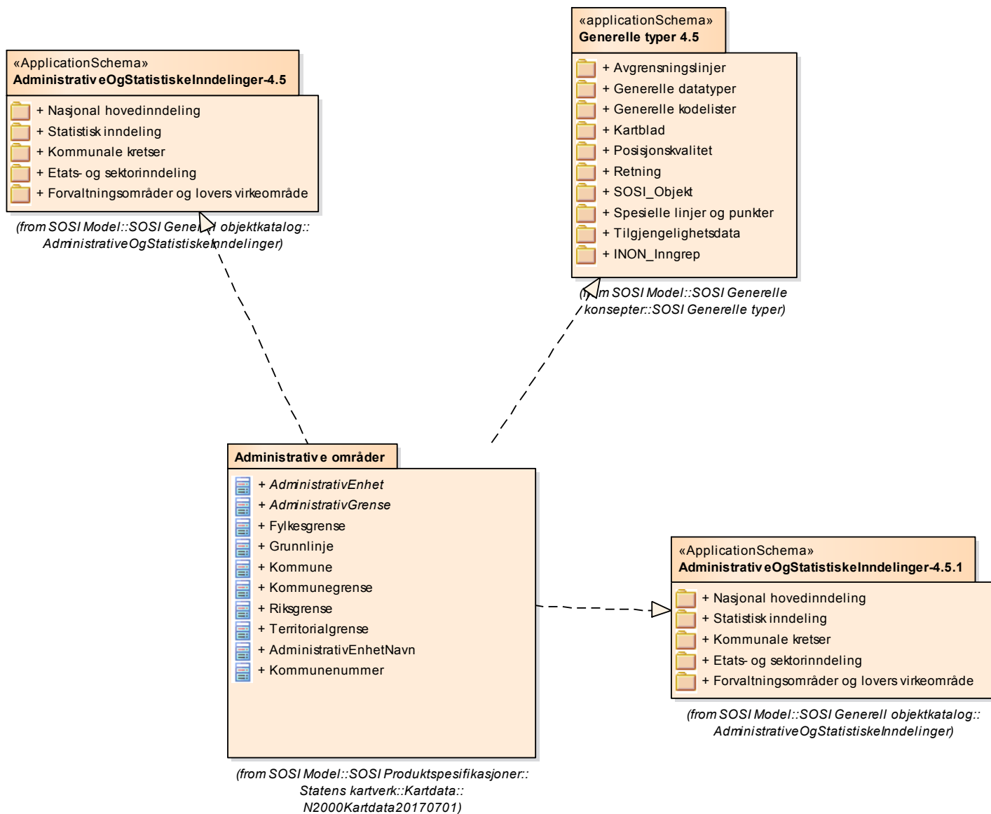
Figur 5 Pakkeavhengighet
