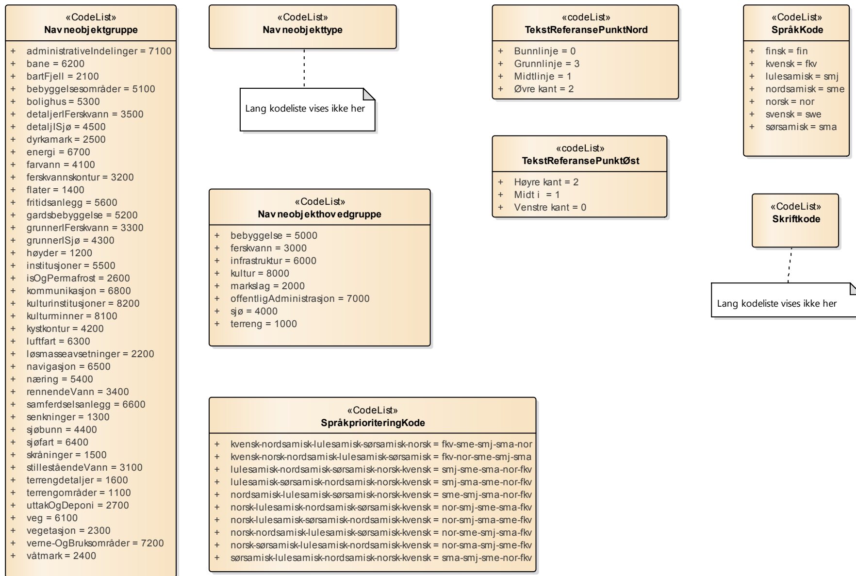
Figur 49 Kodelister
