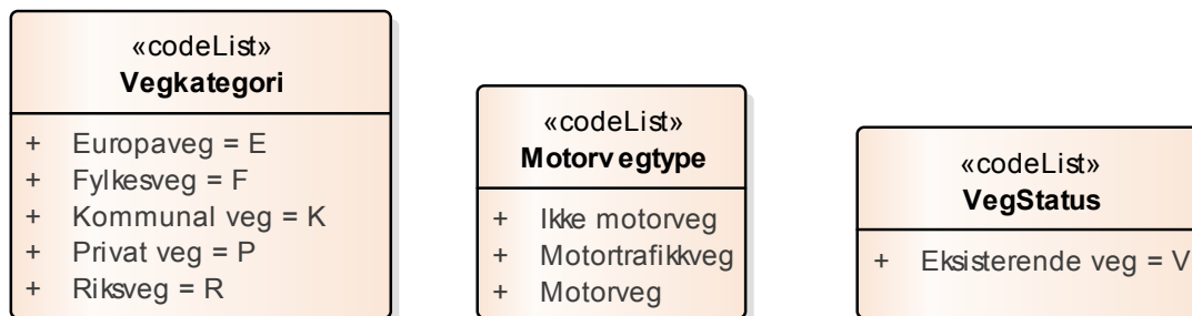
Figur 43 Kodelister
