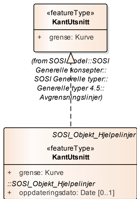
Figur 2 KantUtsnittrealisering
