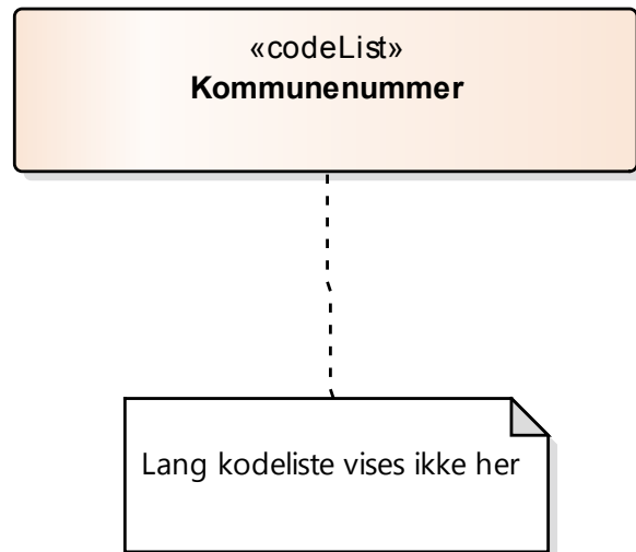
Figur 11 Kodelister
