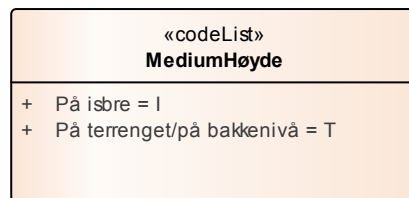
Figur 31 Kodelister
