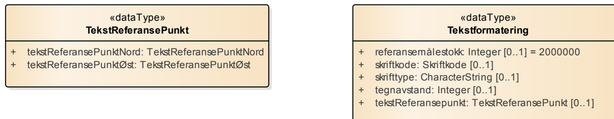
Figur 48 Datatyper
