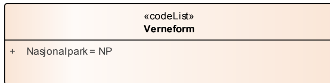
Figur 36 Kodelister
