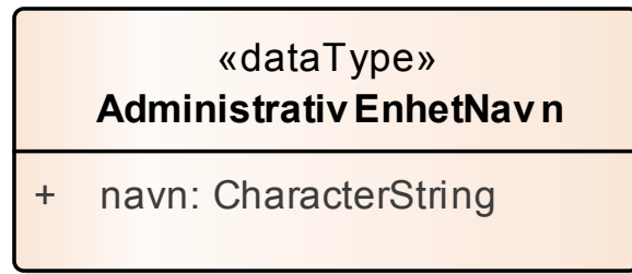
Figur 10 Datatyper
