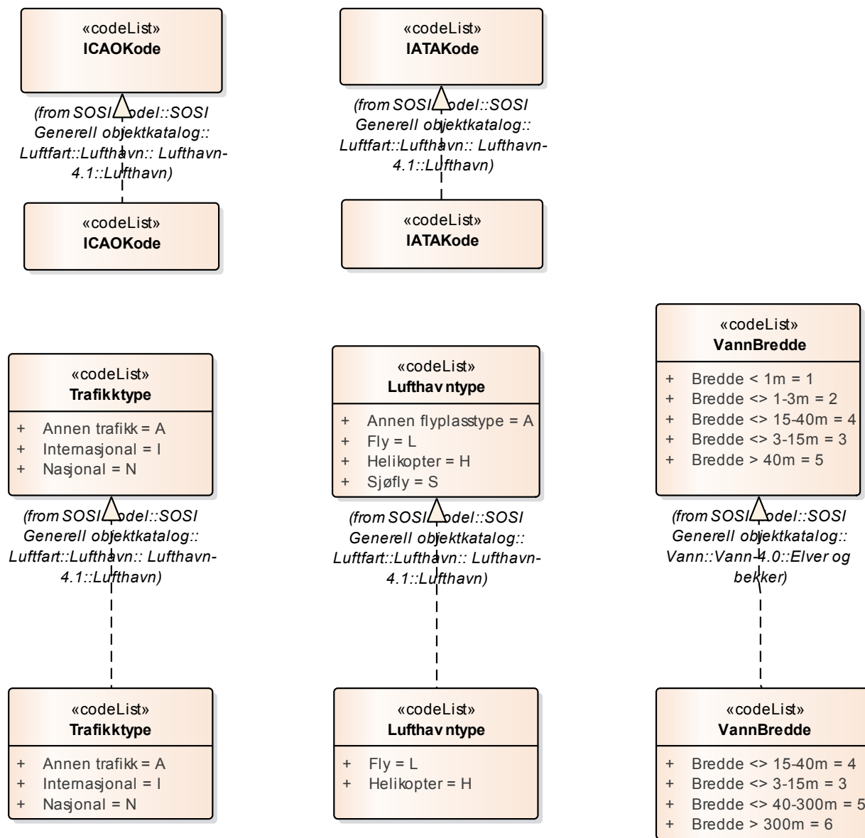
Figur 14 Realisering av kodelister fra generell objektkatalog
