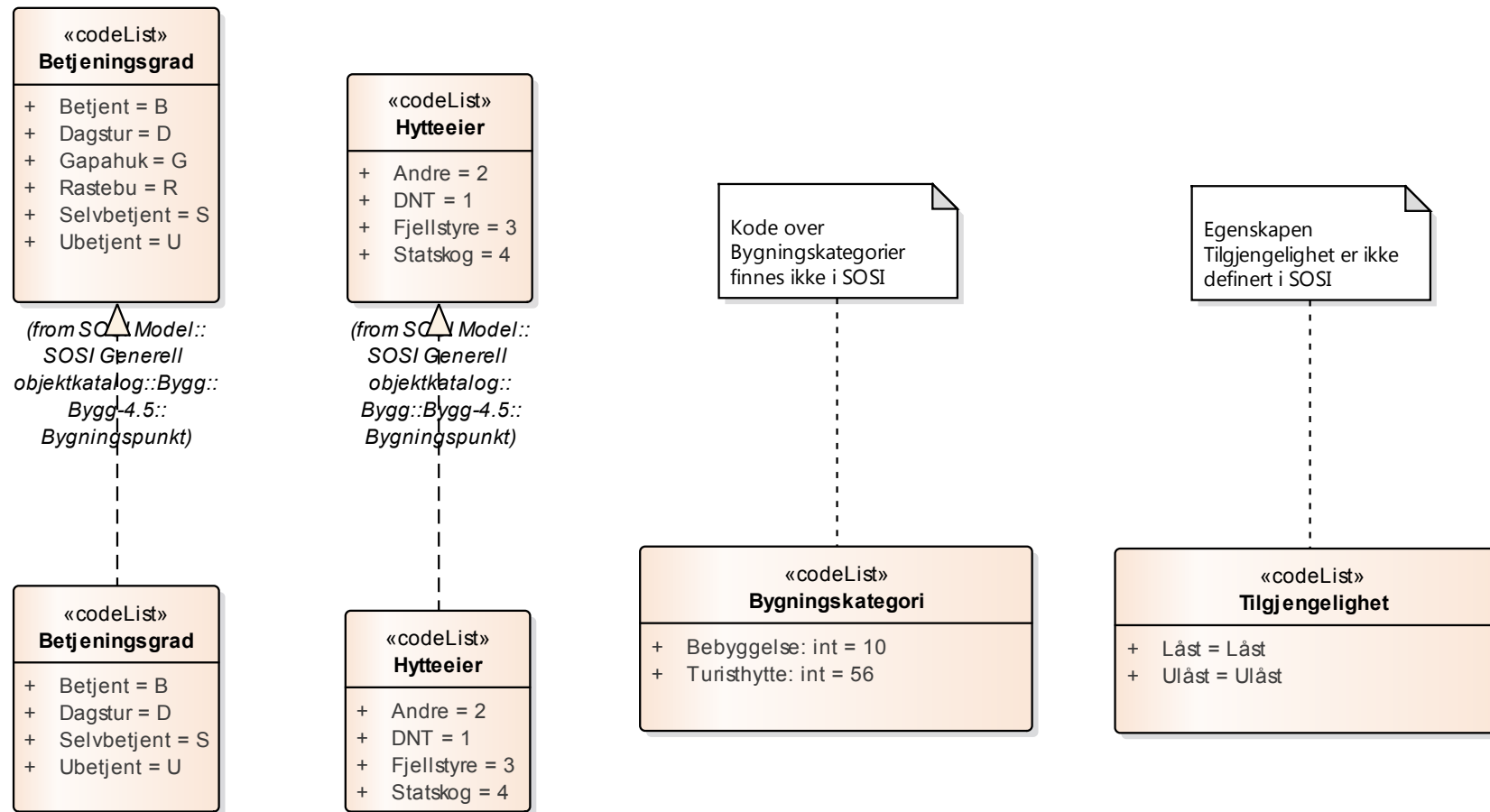
Figur 26 Realisering av kodelister fra generell objektkatalog
