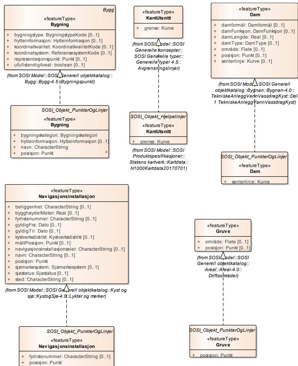
Figur 24 Realisering av featuretyper fra generell objektkatalog
