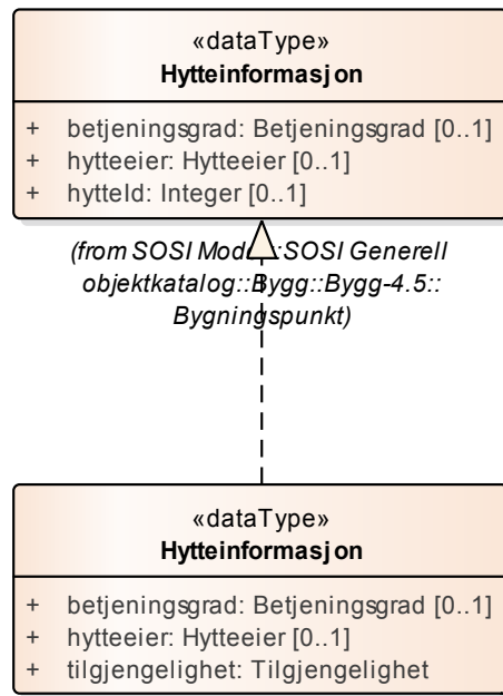
Figur 25 Realisering av datatyper fra generell objektkatalog
