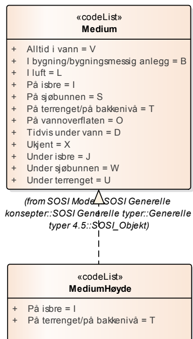
Figur 32 Realisering av kodelister og datatyper fra generell objektkatalog
