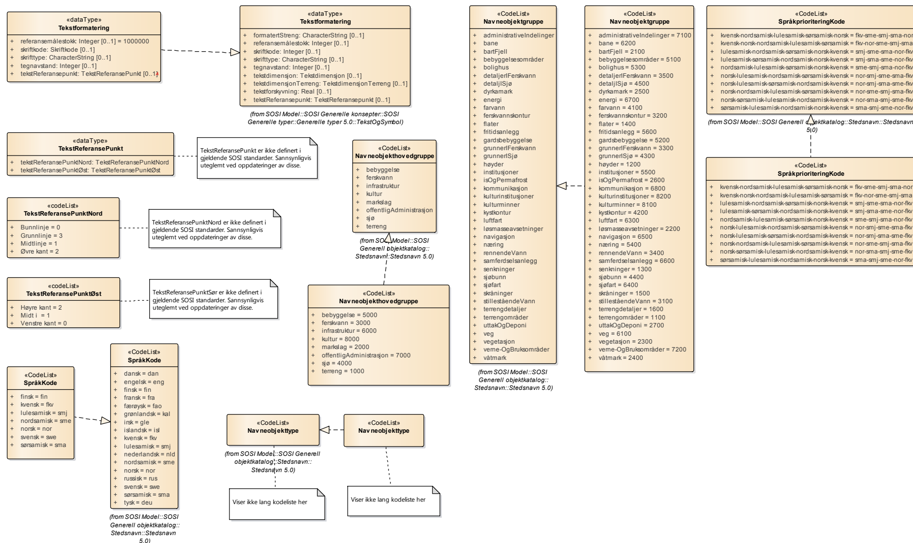
Figur 50 Realisering av datatyper og kodelister fra generell objektkatalog
