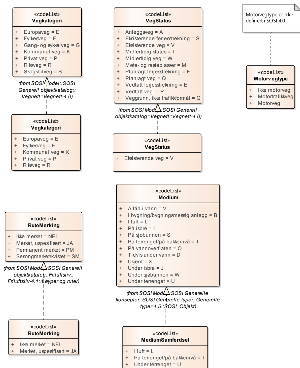
Figur 44 Realisering av kodelister fra generell objektkatalog
