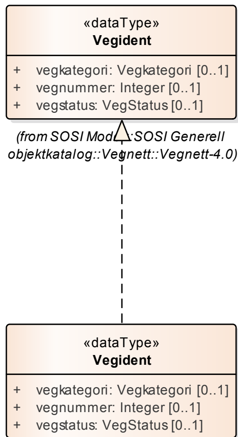
Figur 43 Realisering av datatyper fra generell objektkatalog
