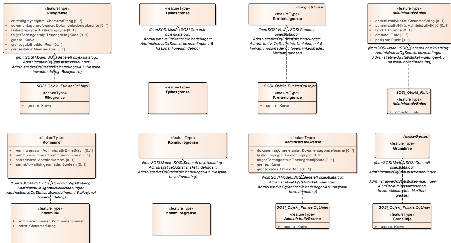
Figur 6 Realisering av featuretyper fra generell objektkatalog
