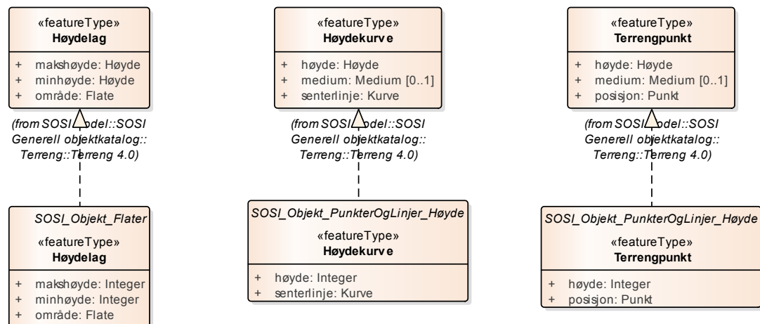
Figur 31 Realisering av featuretyper fra generell objektkatalog
