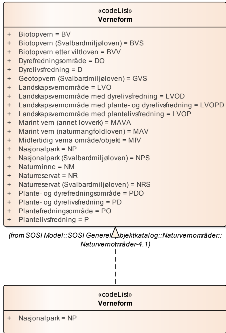
Figur 38 Realisering av kodelister fra generell objektkatalog
