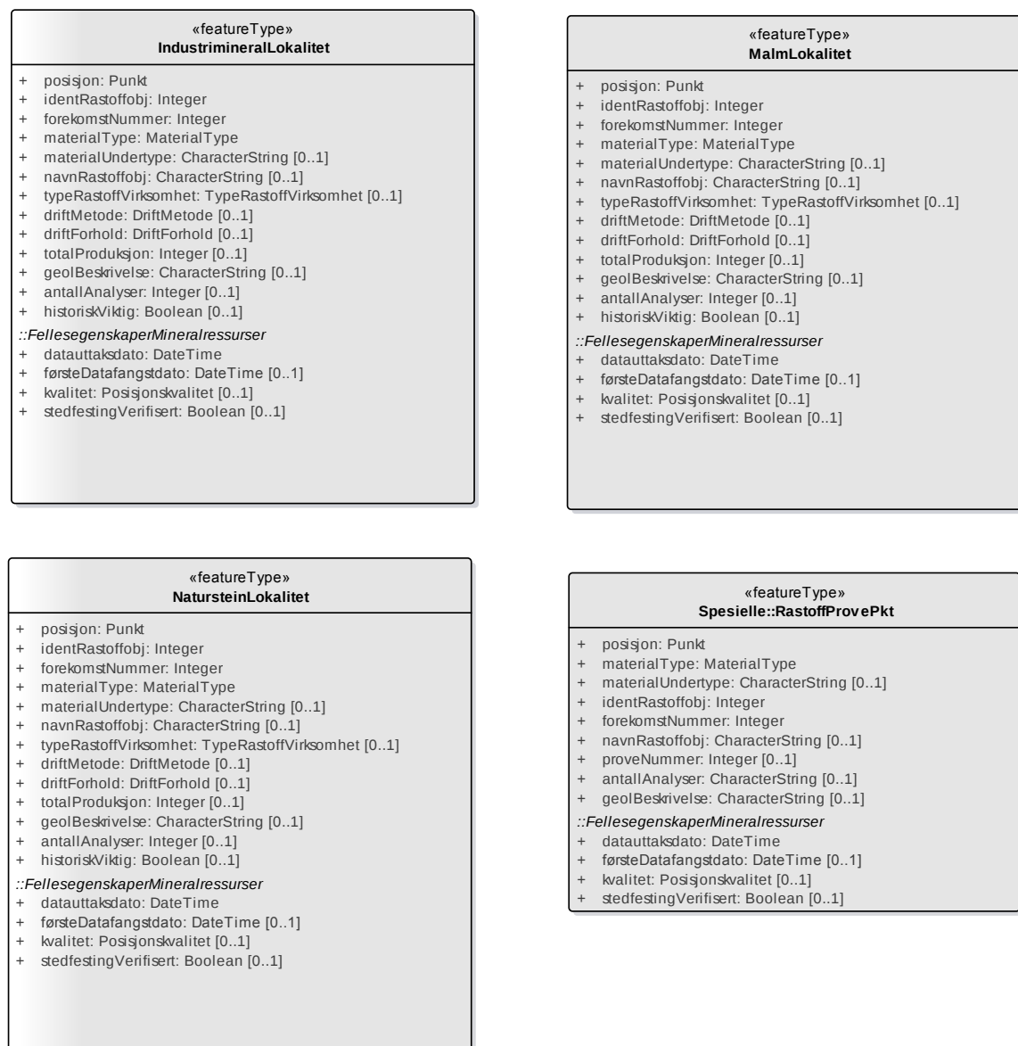
Figur 8 Hovedskjema
