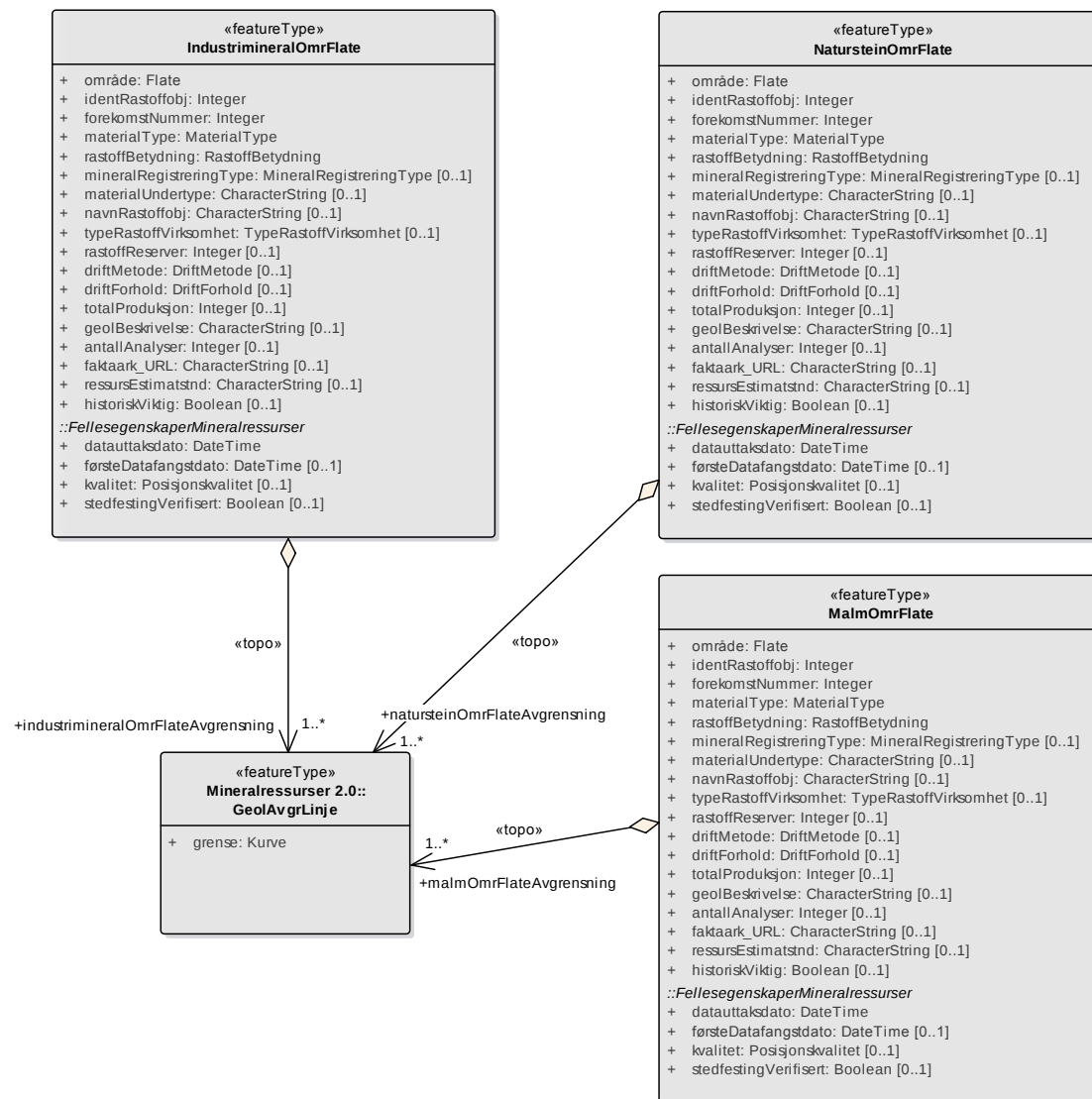
Figur 6 Hovedskjema
