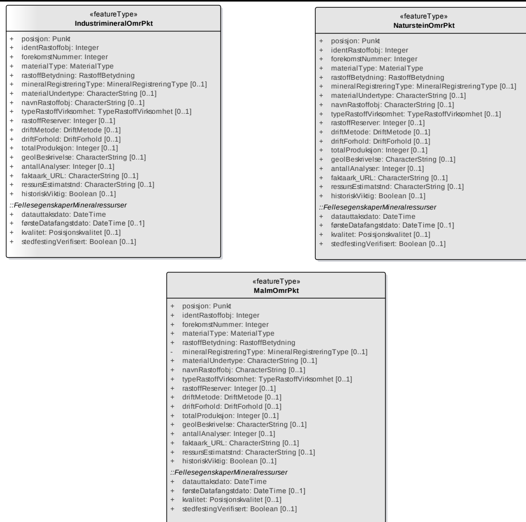
Figur 7 Hovedskjema
