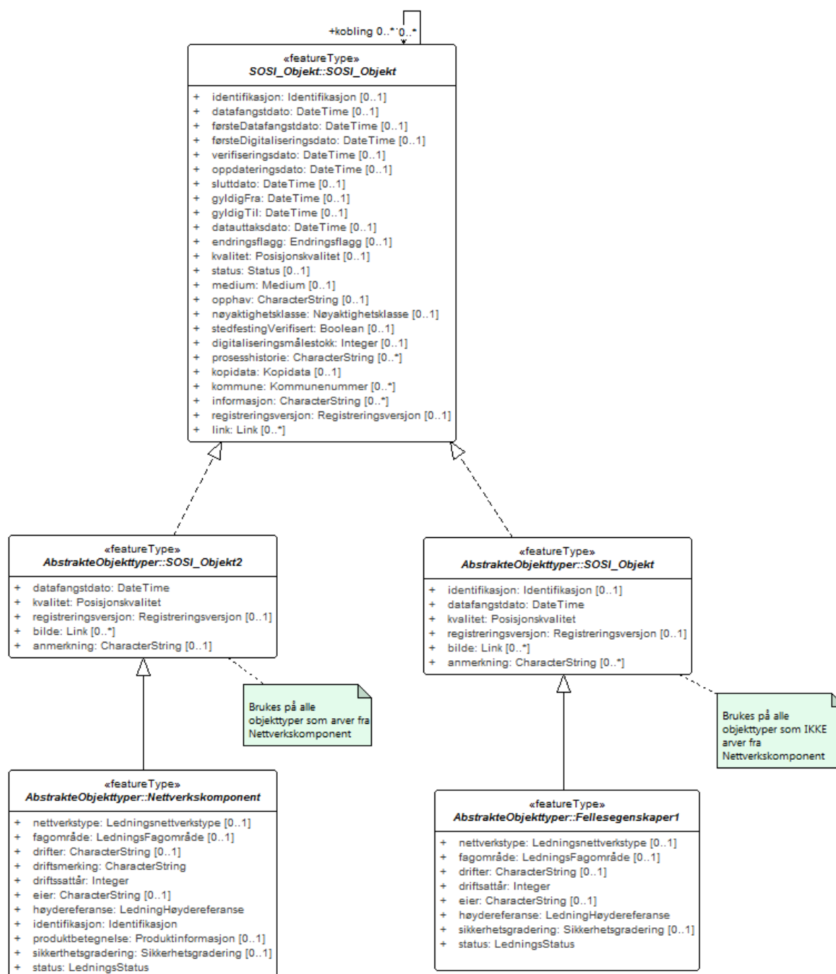
Figur 18 Realisering SOSI_Objekt
