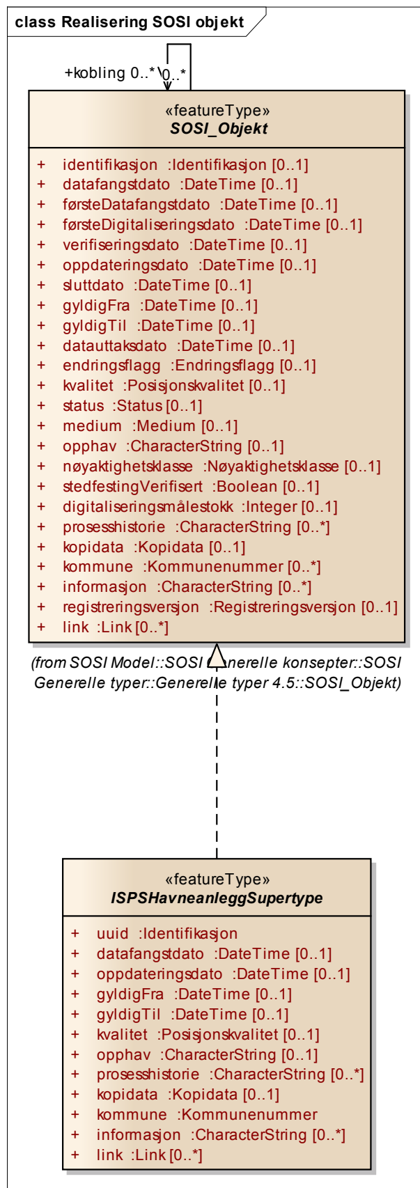
Figur 3 Realisering SOSI objekt
