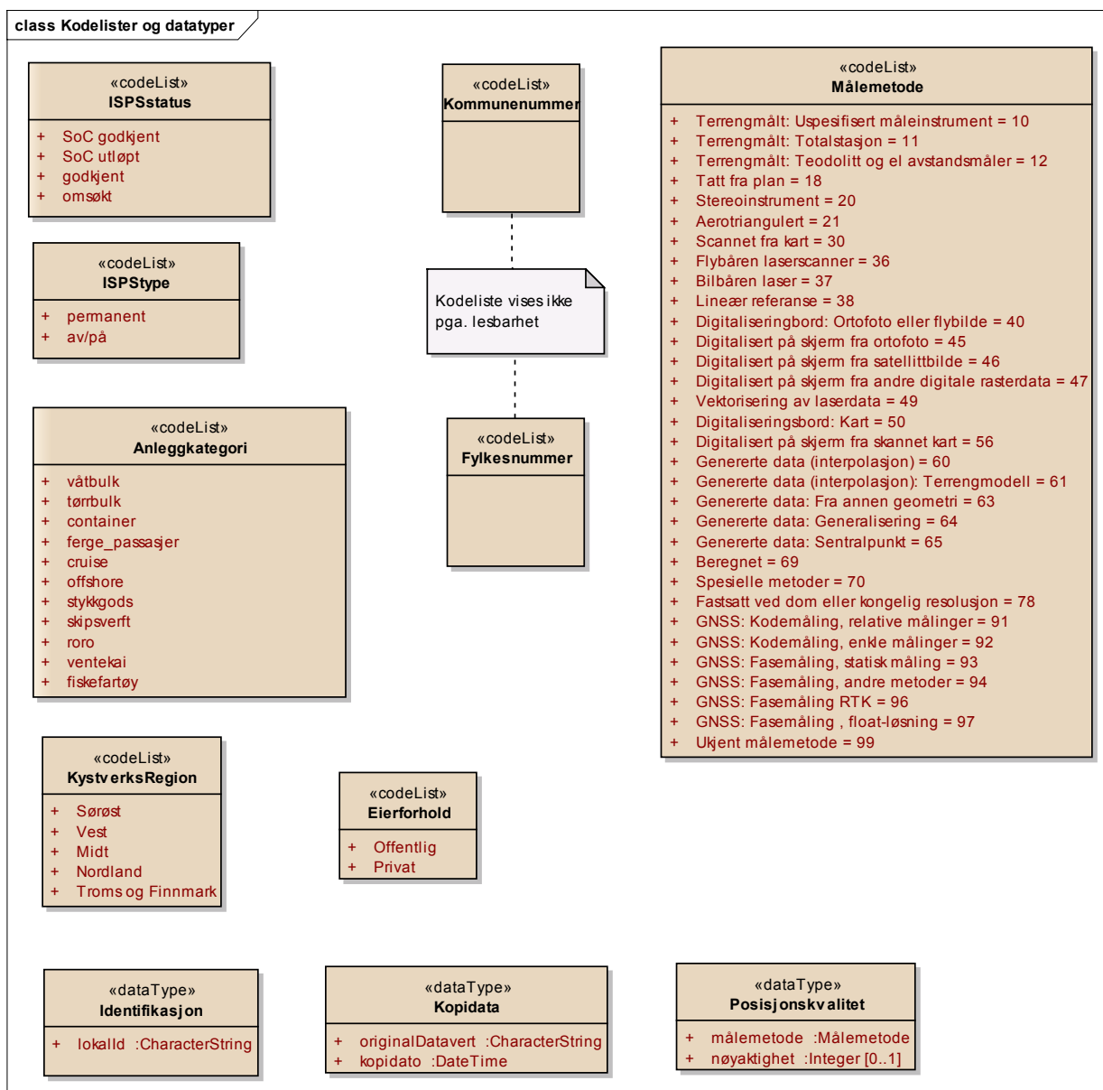
Figur 2 Kodelister og datatyper
