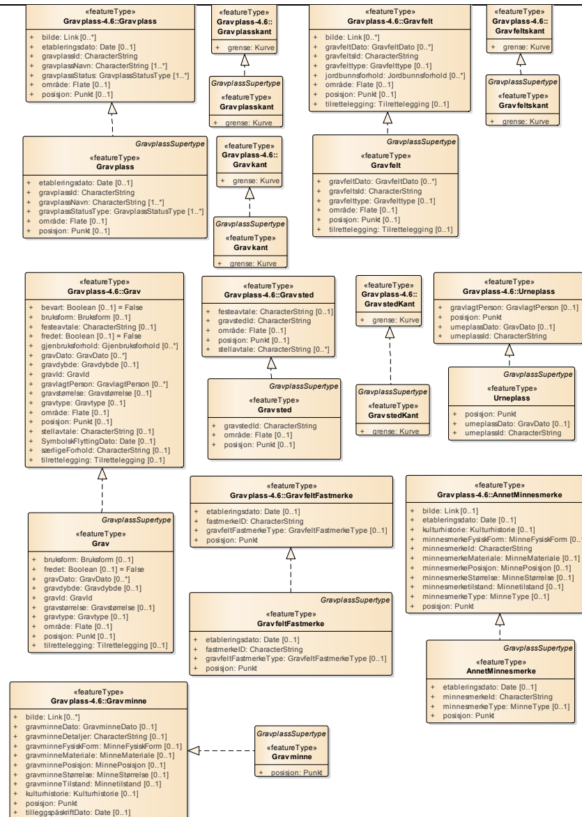
Figur 6: Realisering fra fagområde
