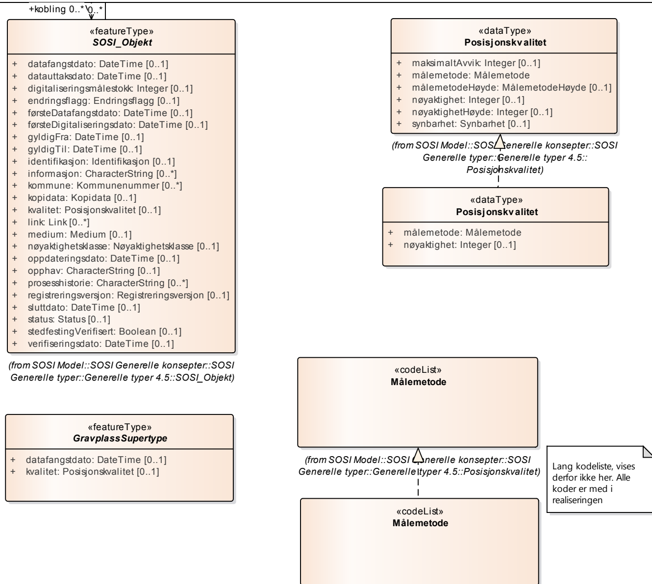
Figur 8: Realisering fra Generelle Typer
