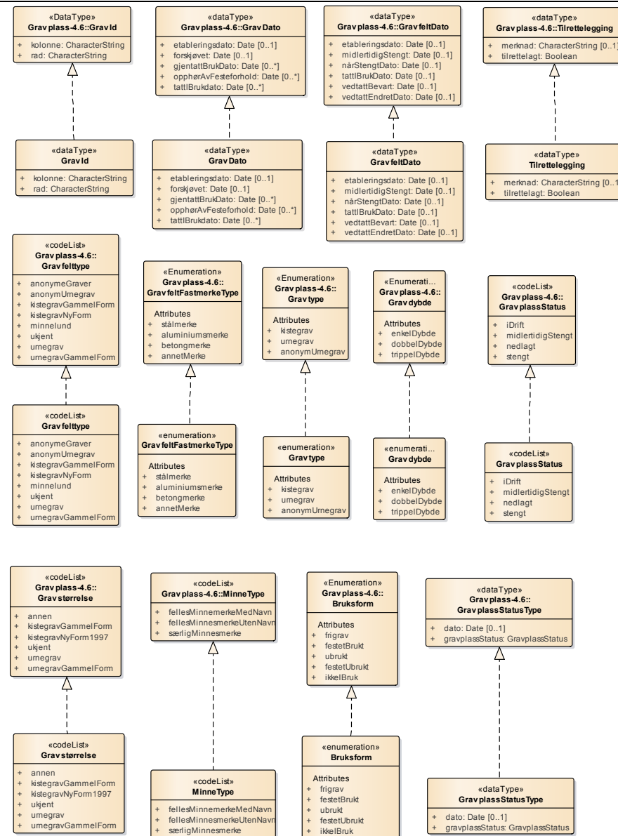
Figur 9: Realisering datatyper og kodelister
