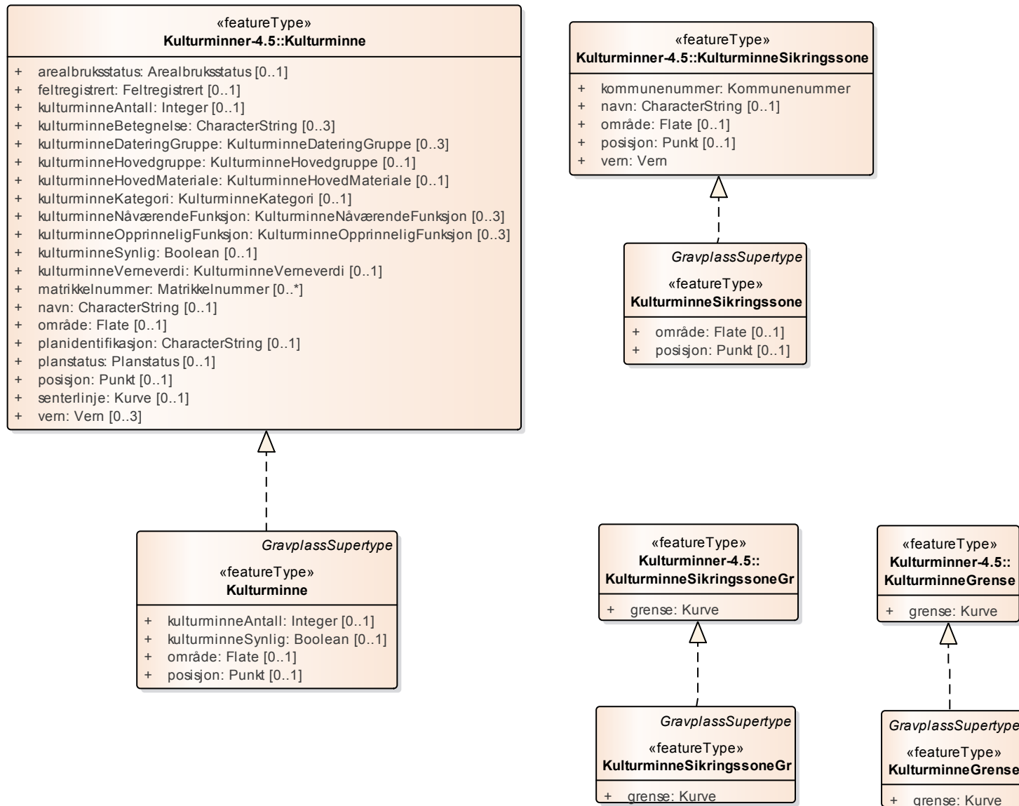
Figur 7: Realisering fra Kulturminne
