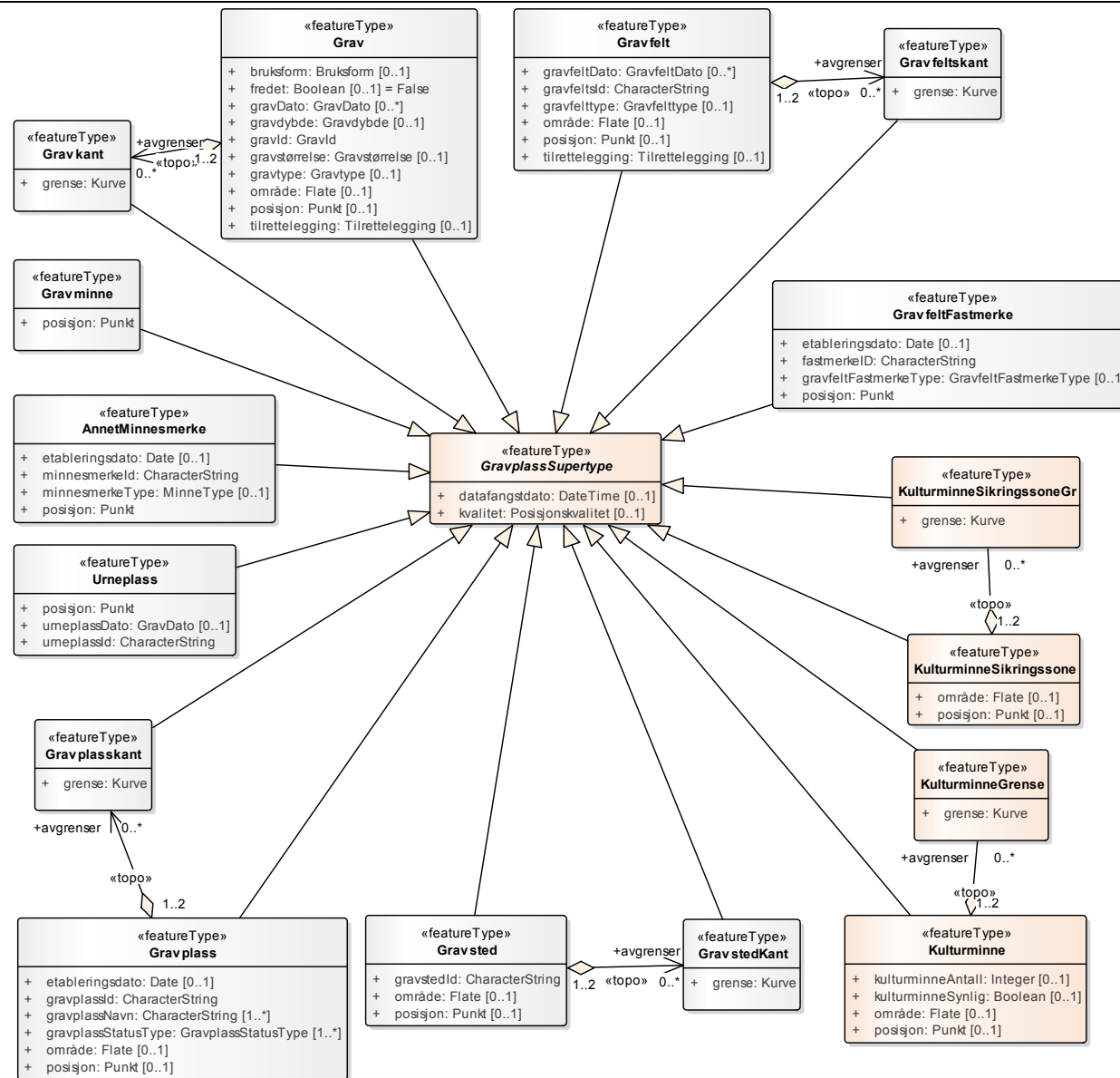
Figur 10: Arv av generelle typer
