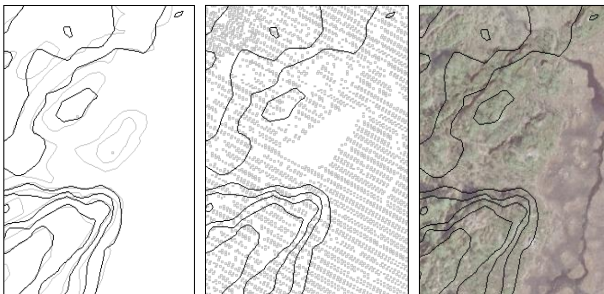
Figur 4 Figuren viser hvordan feil klassifisering av terrengpunkter fører til at en kulle "forsviner" fra terrengmodellen: Grå linjer er fotogrammetrisk konstruert høydekurver, svarte er høydekurver generert fra laserpunktene vist som grå prikker i den midterste figuren. Ortofoto i bakgrunnen viser at vegetasjonen her tilsier at det bør kunne klassifiseres terrengpunkter i området.
