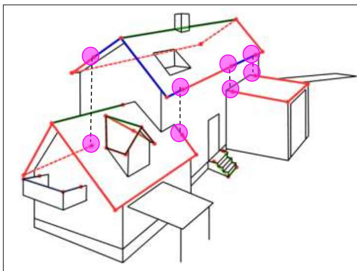
Figur 16. Eksempel på 2D-nodepunkt for en bygning. Disse er markert med en rosa ring. Kilde: Produktspesifikasjon for FKB.
