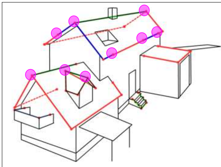
Figur 15. Eksempel på 3D-nodepunkt for en bygning. Disse er markert med en rosa ring. Røde linjer er takkant, mørkeblå linjer er taksprang, brune linjer er bygningslinjer og mørkegrønn linje er mønelinje. Kilde: Produktspesifikasjon for FKB.
