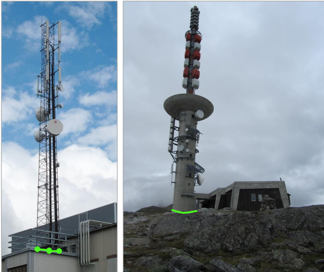
Figur 27: Eksempel på registrering av masteomriss. Hvert enkelt punkt i kurven angir det enkelte fundament for masten.
