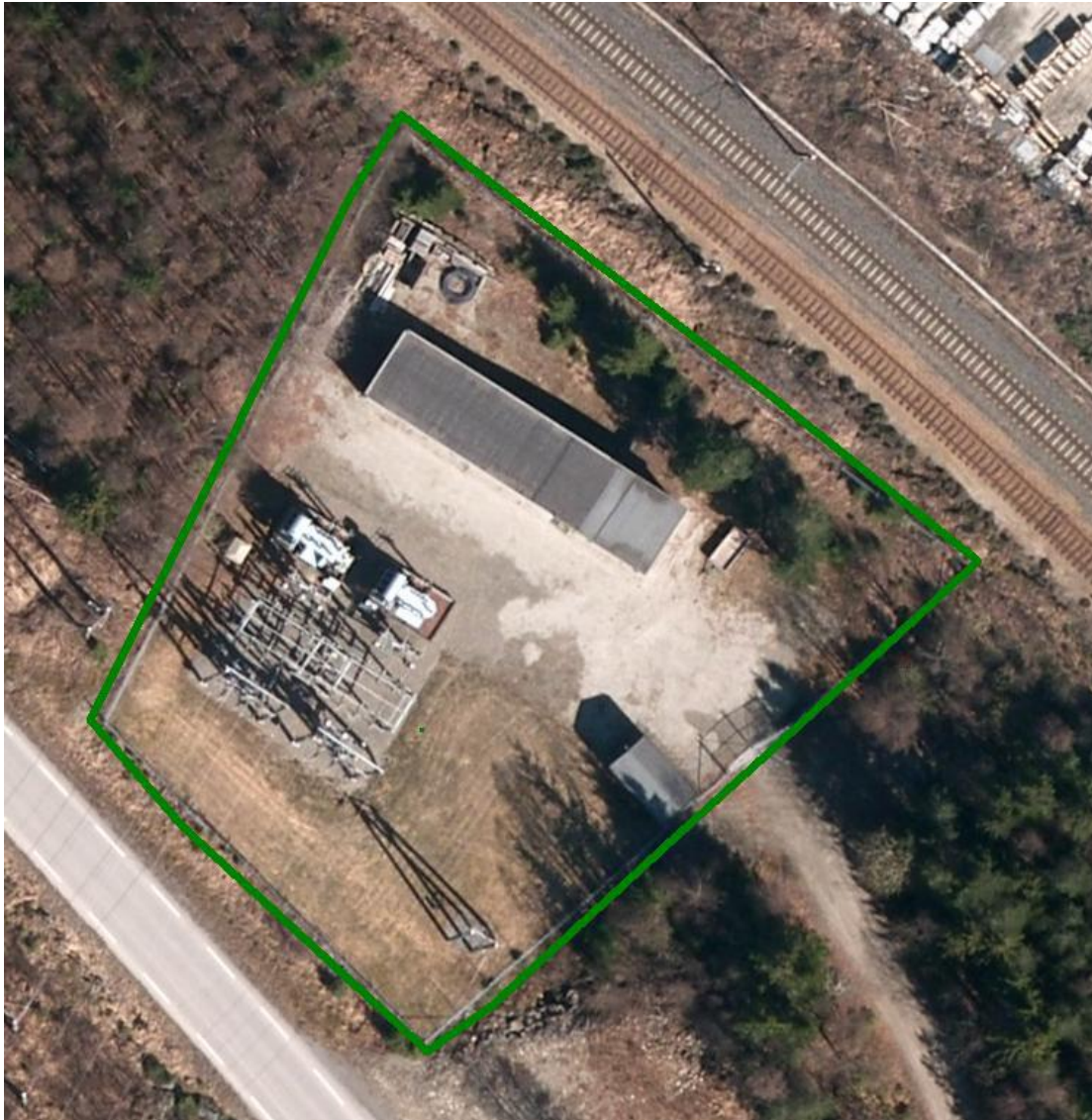
Figur 36: Avgrensing av trafostasjon skal gjøres ved hjelp av arealbruksobjekt IndustriOmråde
